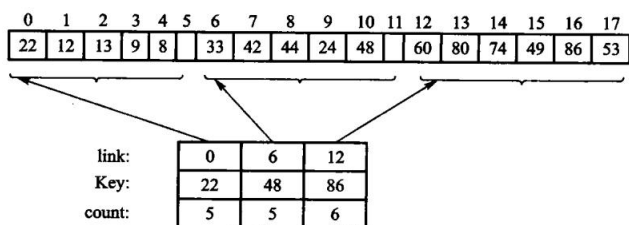
原书图 10.3 把主表分成三块：
