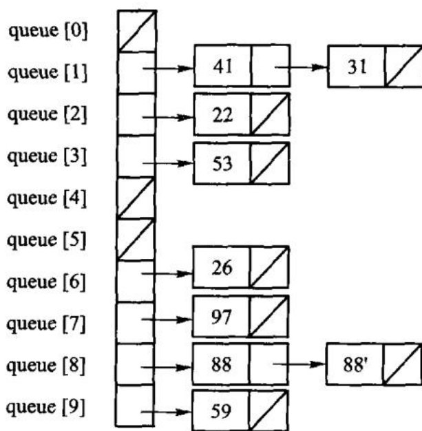
(b) 第一趟分配结果
