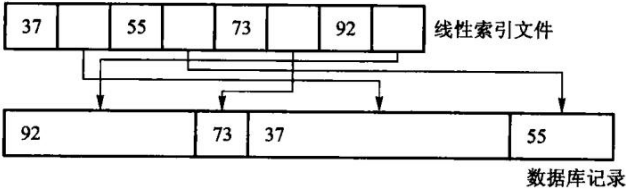
图 11.1 线性索引，图中的数据库记录不等长
