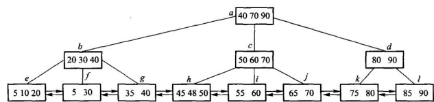
图 11.9 3 阶 B + 树
