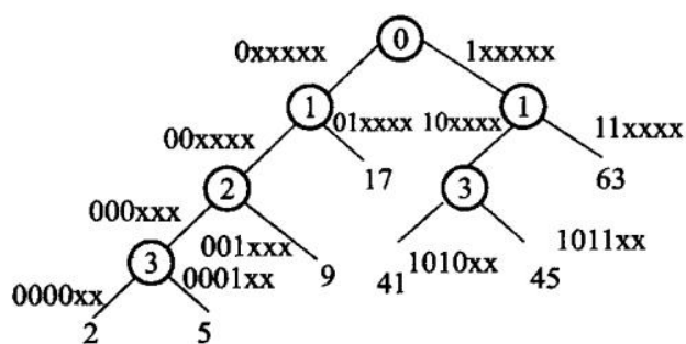
图 12.19 x 表示那个位可以为 1 或者 0
