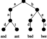
(a) 单词等长
