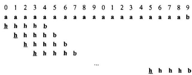
图 4.8 匹配失败的最佳情况示例
