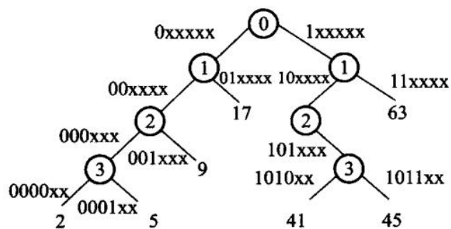
图 12.18 对 Trie 树的改进
