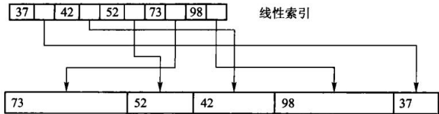
图 1.4 索引示例
