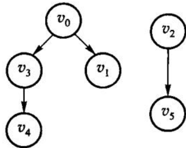
图 7.9 有向图及其生成森林; (b) 有向图的生成森林
