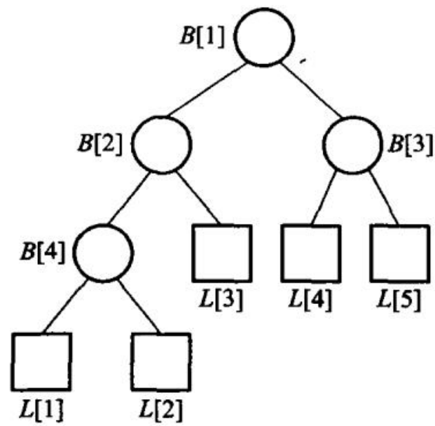
图 9.4 含有 5 个选手的赢者树
