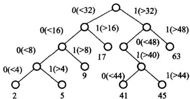
图 12.16 一棵二叉 Trie 树
