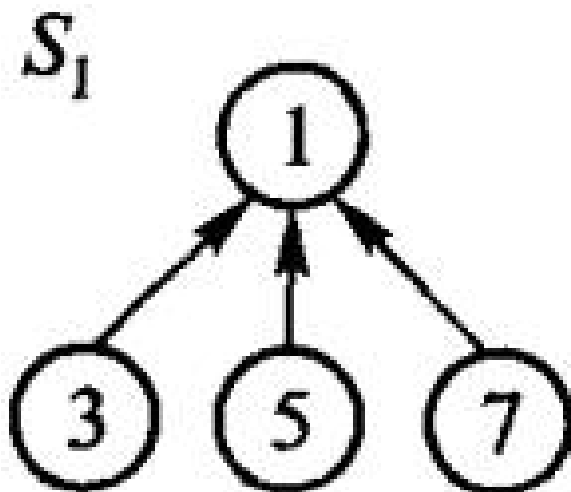
图 6.10 用每个结点的父指针表示树。
