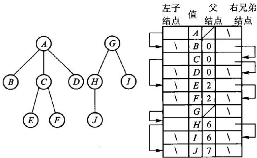
图 6.7 「左子/右兄」表示两棵树 三种周游的访问顺序不同：
