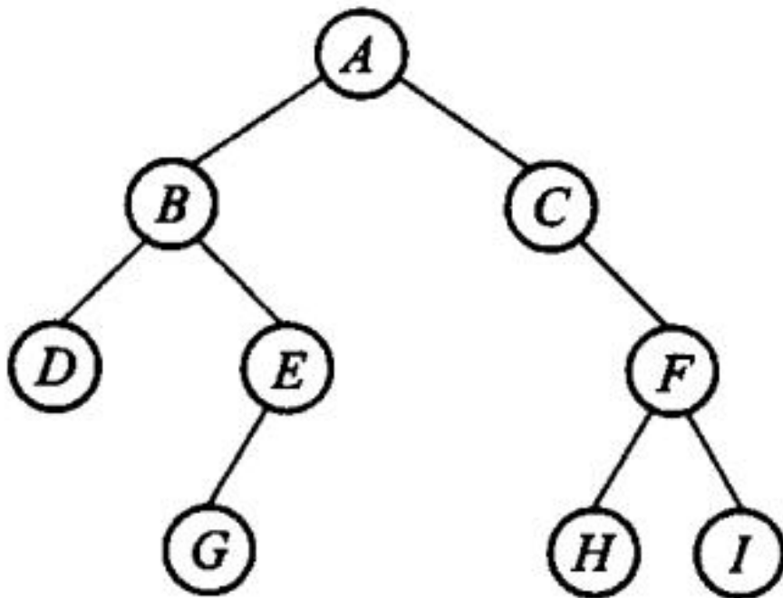
图 5.5 二叉树示例
