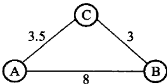
图 7.18 最短路径的示例：从 A 到 B 的最短路径是 A \rightarrow C \rightarrow B ，并不是边数最少的那条。路径上的第一个顶点叫源点 (source)，最后一个是汇点 (sink)。下面两小节分别讨论单源最短路径和每对顶点之间的最短路径。
