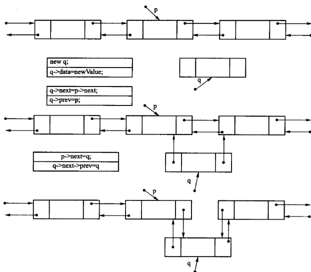
图 2.12 双链表插入操作示意。四条赋值的次序有一处不能反： q \rightarrow next = p \rightarrow next 必须在 p \rightarrow next = q 之前——先改 p \rightarrow next 就丢了原来的后继；而最后一句 q \rightarrow next \rightarrow prev = q 要借 q \rightarrow next 找到后继，也必须排在 q \rightarrow next 填好之后。稳妥的做法就是原书的次序：先让新结点指向两侧，再改两侧指向新结点。
