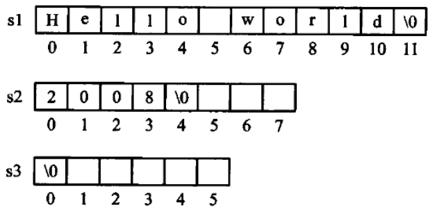
图 4.1 C 风格字符串的变量说明示意。 '\0' 是 ASCII 里 8 位全 0 的 NULL 符，只作结束标记用，不算内容；说明变量时可以用字符串常量给初值，也可以不给——原书说图中的 s3 没给初值，「意味着它存储空字符串」。这只对全局或 static 数组成立（它们会被零初始化）；写在函数里的局部数组不给初值，内容
