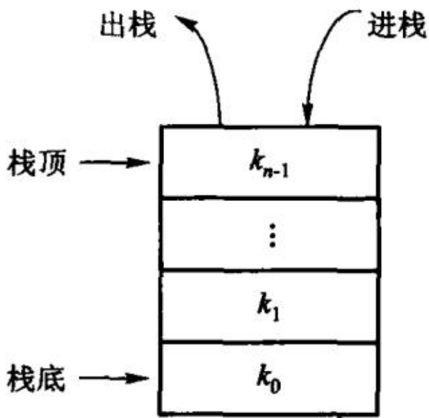
图 3.1 栈的示意图
