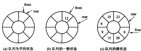
图 3.12 牺牲一格的循环队列（8 格数组最多放 7 个元素）：(a) 空，front == rear；(b) 一般状态；(c) 满， (rear + 1) \% (n + 1) == front 。
