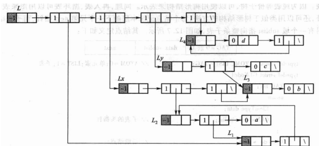
图 12.9 带头结点的循环广义表。
