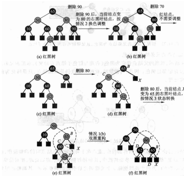
图 11.25 连续删除 90、70、80 引起的双黑调整全过程。
