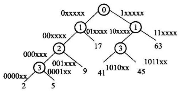
图 12.19 压缩的依据：x 表示该位取 0 取 1 都落在同一枝里，也就是这一位不需要用来分支——把这样的层去掉就是 Patricia。
