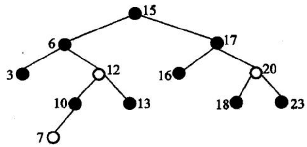
图 11.31 红黑树
