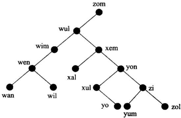
图 12.21 按 K 的给定次序插入得到的二叉搜索树。
