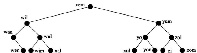
图 12.24 最佳二叉搜索树
