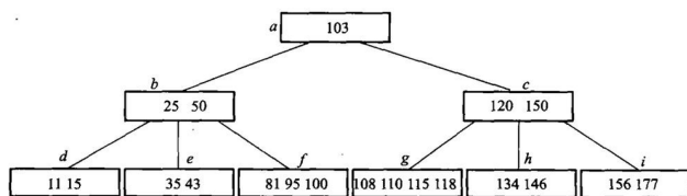
(a) 5阶B树
