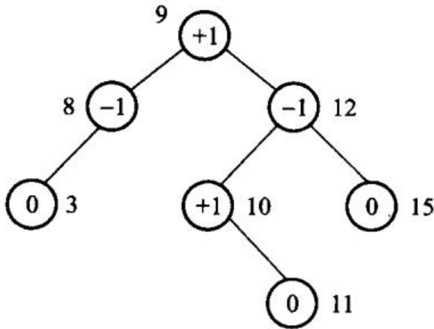
图 12.29 带平衡因子的 AVL 树。实现时结点里存的不是高度而是这个因子，只要两
