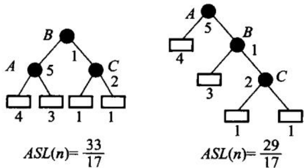
图 12.26 结点权不等时，最佳的形状未必最平衡：权大的关键码要往根靠，哪怕整棵树因此歪一些。这正是需要动态规划、而不是简单「取中位数当根」的原因。
