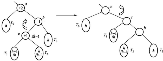
(b) 中间状态平衡因子无意义
