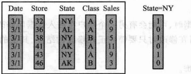
(a) 百货销售数据库记录以及 State=NY（纽约州）的位向量
