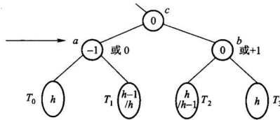
(c) a的平衡因子为-1或0, b的平衡因子为0或+1
