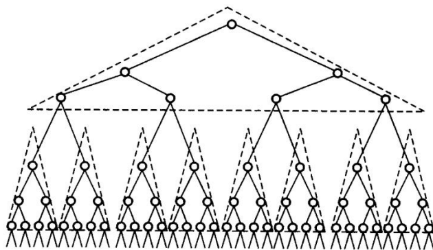
图 11.3 多分树
