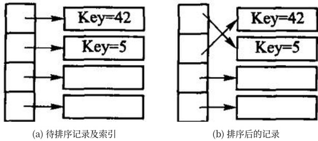
图 8.13 索引排序示意: (a) 待排序记录及索引; (b) 排序后——记录一个都没动, 动的是索引。
