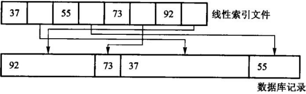
图 11.1 线性索引，图中的数据库记录不等长
