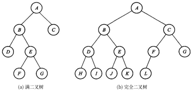
图 5.2 (a) 满二叉树；(b) 完全二叉树。
