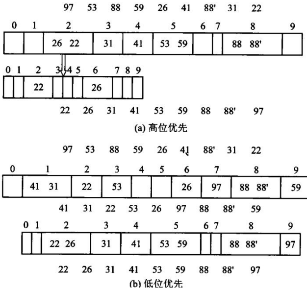
(b) 低位优先; 图 8.10 基数排序
