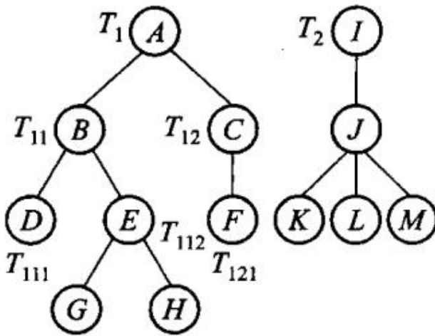
(a) 由 T_1 T_2 构成的森林
