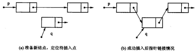
图 2.7 插入示意：新结点的 next 先接上前驱原来的后继（图中的 \square ），再把前驱的 next 改指向新结点（ \square ）。两步的次序不能反——先改前驱就再也找不到原来的后继了。
