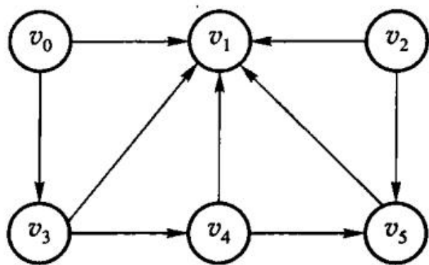
(a) 有向图
