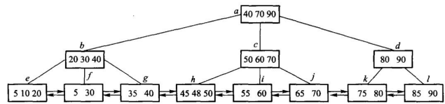
图 11.9 3 阶 B + 树
