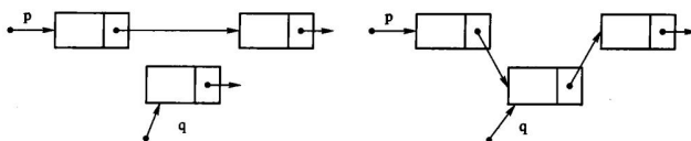
(a) 准备新结点，定位待插入点
