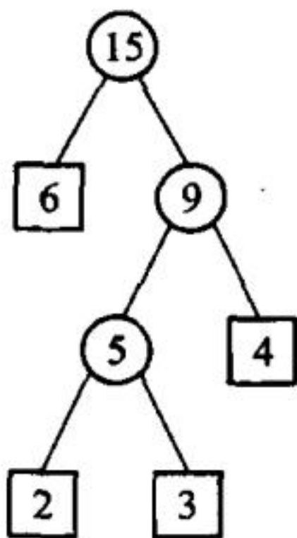
图 5.19 Huffman 树的构造过程
