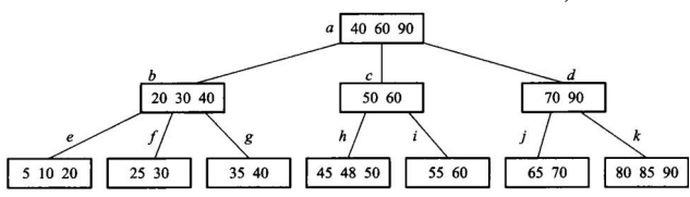
图 11.11 从图 11.9 的 3 阶 B + 树中删除 75 后
