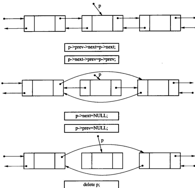
图 2.11 双链表的删除操作示意
