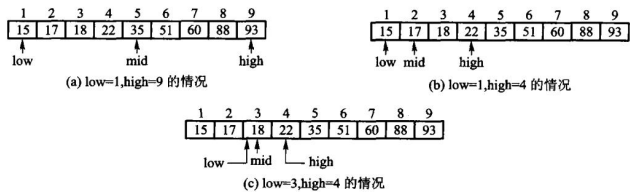
图 10.1 二分检索 K = 18 的过程
