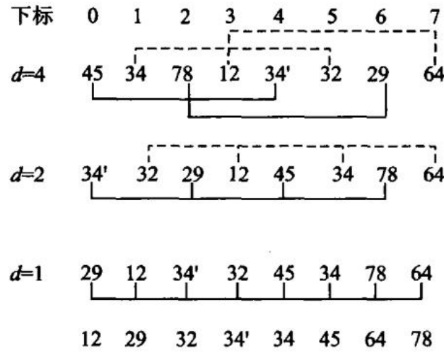
图 8.2 Shell 排序
