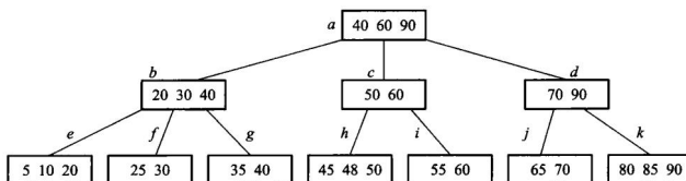
图 11.11 从图 11.9 的 3 阶 B+ 树里删掉 75 之后。内部结点上那份 75 的复写可以留
