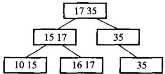
图 11.29 2 阶 B^+ 树图示
