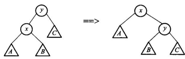
图 12.38 只有当被展开的结点已经是根的孩子时，才做单旋转：左边是旋转前，右边是旋转后。
