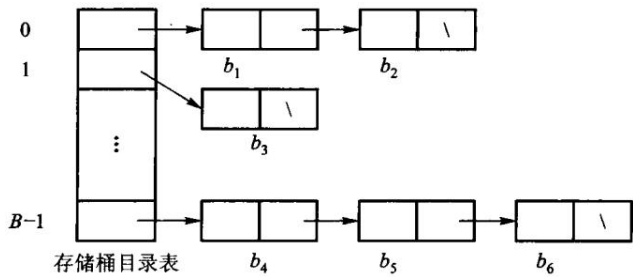
图 10.8 具有 B 个存储桶的散列文件组织。存储桶目录表存 B 个指针，各指向对应桶的第一个页块；1 号桶只有一个页块， B - 1 号桶由 b_4 、 b_5 、 b_6 三块串成，每桶最后一块的指针为空。检索一次要一次访外读目录表、再逐块查桶，平均访外次数约为桶内页块数的一
