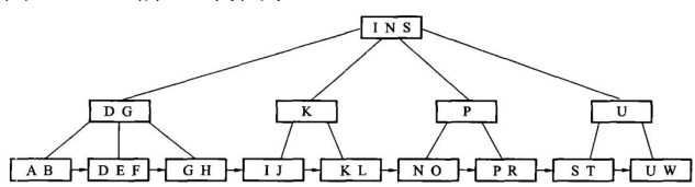
图 11.30 混合型 B^+ 树，内部结点阶为 4、叶结点阶为 3
