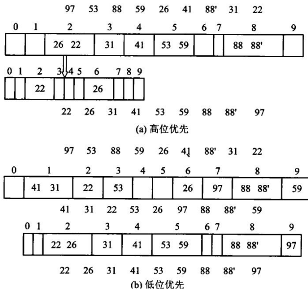
(b) 低位优先; 图 8.10 基数排序
