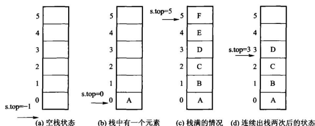
图 3.3 顺序栈的存储结构：(a) 空栈， \text{s.top} = -1 ；(b) 栈中有一个元素， \text{s.top} = 0 ；(c) 栈满， \text{s.top} = \text{mSize} - 1 ；(d) 在 (c) 上连续出栈两次之后。
