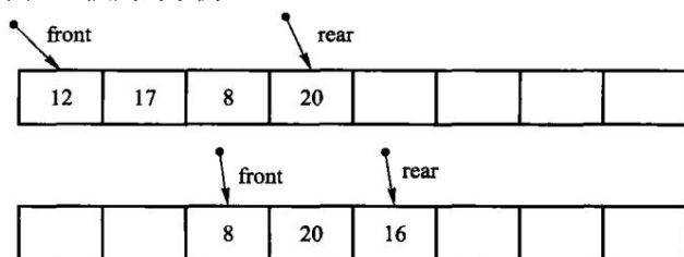
图 3.10 顺序队列的实现示意
