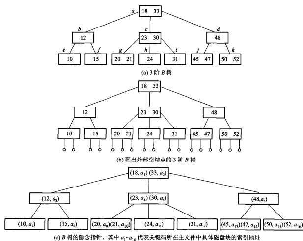
图 11.5 同一棵 3 阶 B 树的三种画法: (a) 通常的画法; (b) 把外部空结点画出来; (c) 画出隐含指针—— a_1 \sim a_{16} 是关键词在主文件里对应磁盘块的索引地址。B 树的关键码在内部结点上带着数据地址, 这正是它与后面 B+ 树的分水岭。
