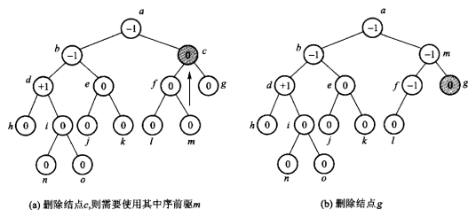
图 12.35 删除之后的调整。删除比插入麻烦：插入最多转一次就结束，删除可能一路向上每层都要转。
