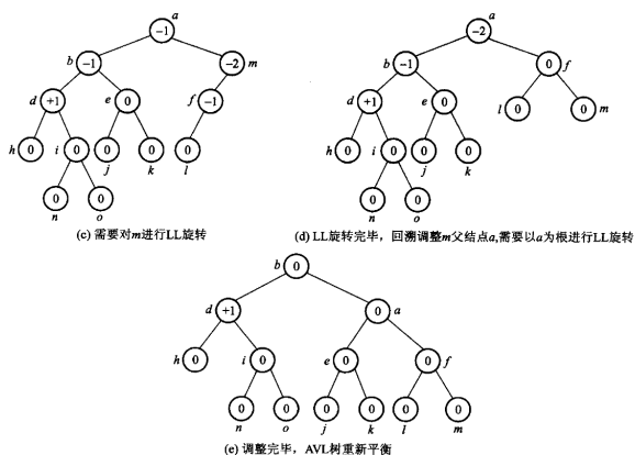
图 12.36 删除的例子（原书跨两页，(a)(b) 一页、(c)(d)(e) 一页）：(a) 删有两个孩子的结点 c ，先用它的中序前驱 m 顶替，再删到叶那一层；(b) 删结点 g 之后 m 失衡；(c) 需要对 m 作 LL 旋转；(d) 转完 m 之后回溯，父结点 a 又失衡，再以 a 为根作一次 LL 旋转；(e) 调整完毕，整棵树重新平衡。一次删除可能引发从被删结点一路到根的多次旋转，这是它与插入最大的不同。
