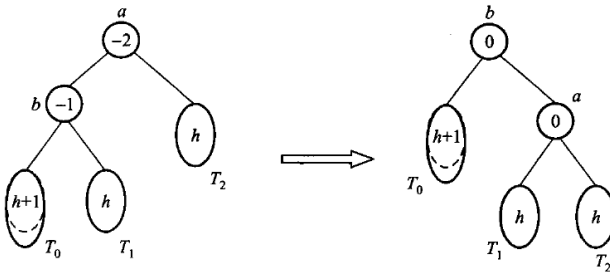
图 12.32 LL 型失衡的单旋转, RR 型对称。
