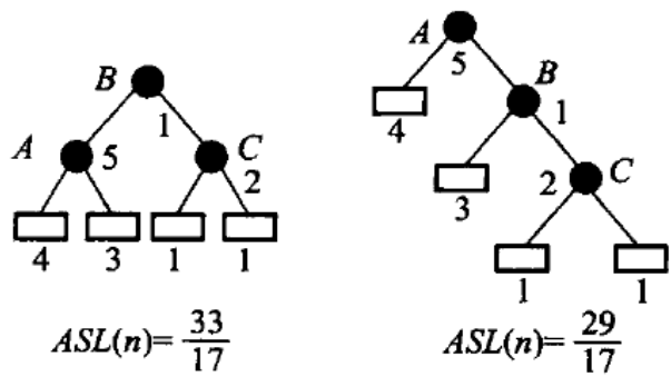
图 12.26 结点权不等时，最佳的形状未必最平衡：权大的关键字码要往根靠，哪怕整棵树因此歪一些。这正是需要动态规划、而不是简单「取中位数当根」的原因。
