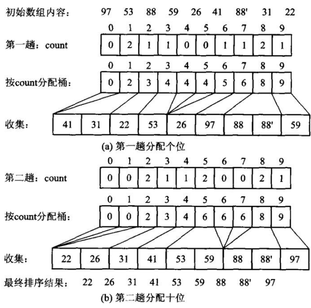
图 8.11 基于顺序存储和桶排序的基数排序
