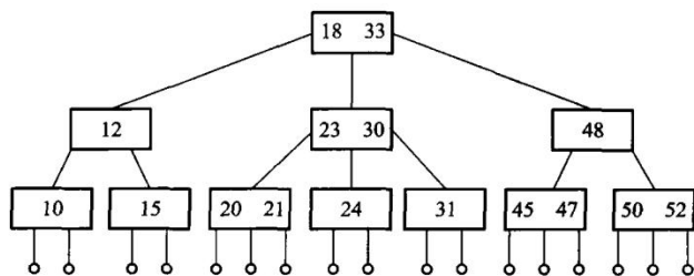
(b) 画出外部空结点的 3 阶 B 树
