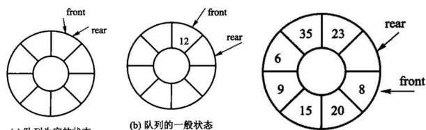
图 3.12 牺牲一格的循环队列（8 格数组最多放 7 个元素）：(a) 空， \text{front} == \text{rear} ；(b) 一般状态；(c) 满， (\text{rear} + 1) \% (n + 1) == \text{front} 。
