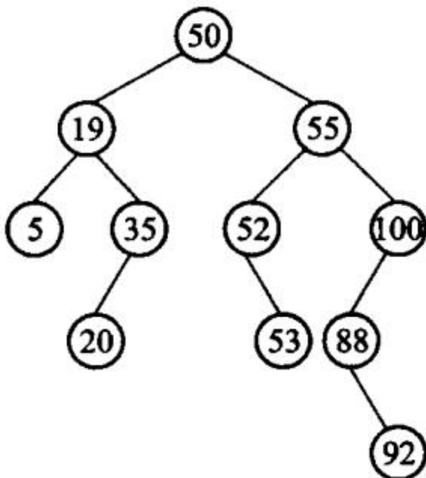
图 5.11 二叉搜索树。检索 key 时把它与根比较：小于就只找左子树，大于就只找右子树，每一步都能扔掉一整棵子树——这就是它比无序线性表快的原因。走到空子树还没找到，
