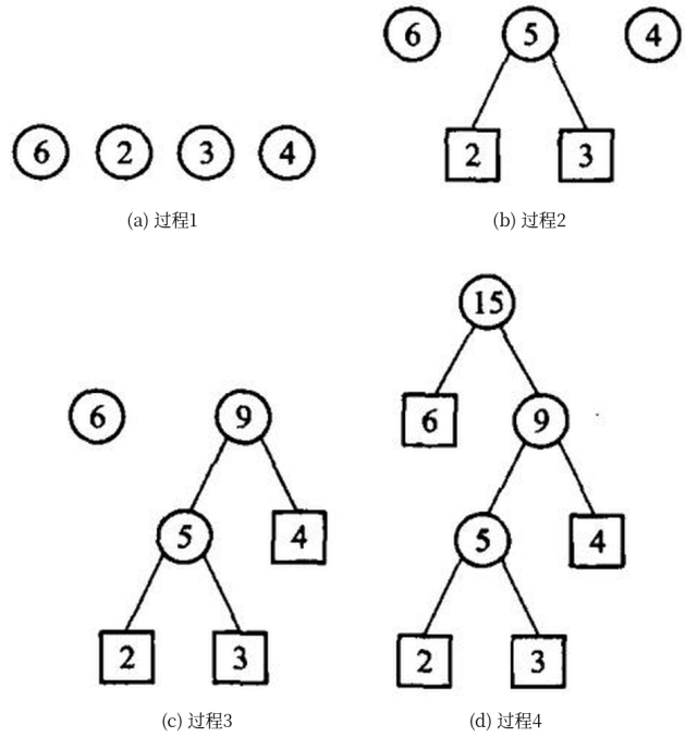
图 5.19 Huffman 树的构造过程： n 个权各自成为一棵单结点树；每次挑出根权最小的两棵，合成一棵新树、新根的权是两者之和；重复 n - 1 次，集合里只剩一棵。
