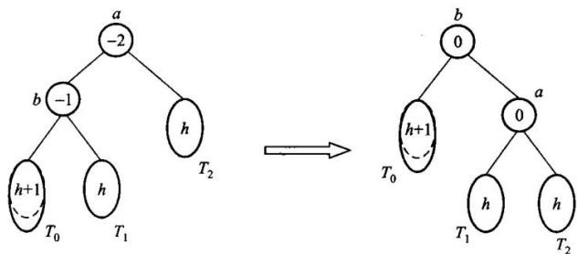
图 12.32 LL 型失衡的单旋转，RR 型对称。
