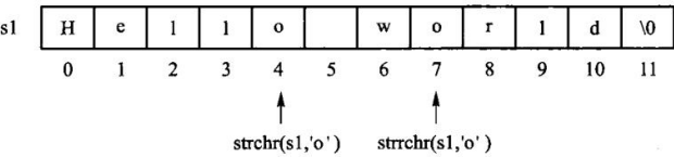
图 4.2 在字符串 s1 中定位字符 ‘ o ’。两个函数返回的都是指针，指向找到的那个字符；找不到返回空指针。本书的 String 用下标和 std::optional 表达同一件事——「没找到」不再靠一个特殊指针值来表示。
