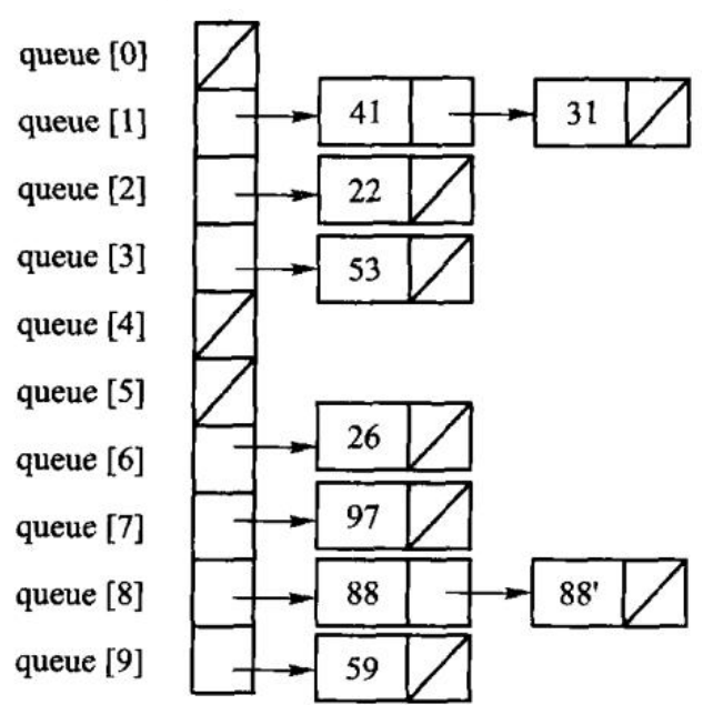
(b) 第一趟分配结果
