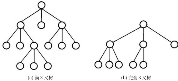
图 6.18 K = 3 时的 (a) 满 3 叉树与 (b) 完全 3 叉树。 K 叉树的分支结点孩子数是定死的，所以链式和顺序两种存法都好实现；完全 K 叉树按编号存进数组，和完全二叉树是同一套办法。计算机图形学里的 4 叉树、8 叉树就是常见的应用。
