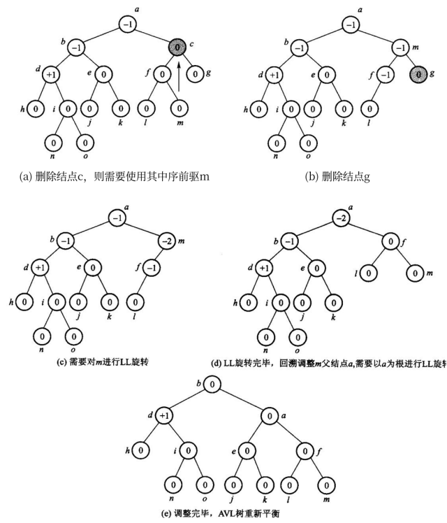
图 12.36 删除的例子：(a) 删有两个孩子的结点 c ，先用它的中序前驱 m 顶替，再删到叶那一层；(b) 删结点 g 之后 m 失衡；(c) 需要对 m 作 LL 旋转；(d) 转完 m 之后回溯，父结点 a 失衡，需要以 a 为根进行 LL 旋转；(e) 调整完毕，AVL 树重新平衡
