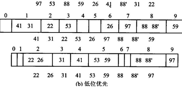
(b) 低位优先; 图 8.10 基数排序
