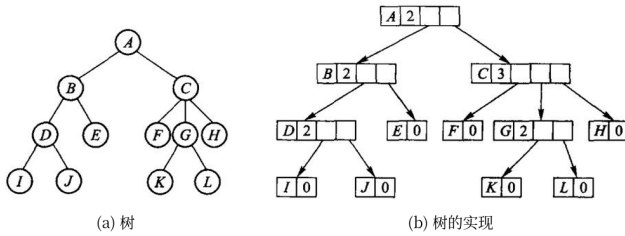
图 6.9 树的动态表示法: (a) 的每个结点在 (b) 里都是一块单独分配的空间, 里面存着孩子数和一张长度可变的孩子指针表。
