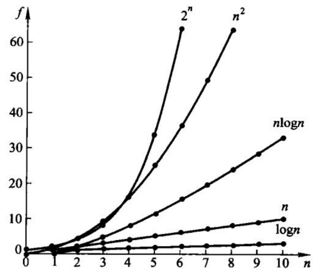
图 1.5 常用函数的增长趋势
