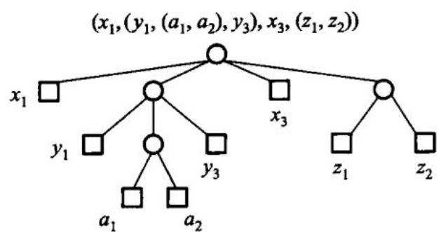
图 12.4 纯表的树表示
