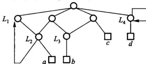
图 12.6 循环表可以看到这是一个有环图；图 12.6 中，因为 L_1 和 L_4 调用自身，导致了回路。其他没有箭头的边，方向都是从上至下的。循环表也可以算作一种存在回路的特殊再入表。
