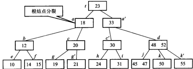
图 11.7 在图 11.5 的 3 阶 B 树中插入键码 19 后导致根分裂
