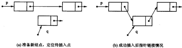
图 2.7 插入示意：新结点的 next 先接上前驱原来的后继（图中的 ），再把前驱的 next 改指向新结点（ ）。两步的次序不能反——先改前驱就再也找不到原来的后继了。
