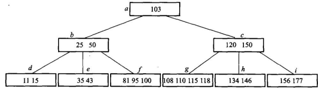
(a) 5 阶 B 树
