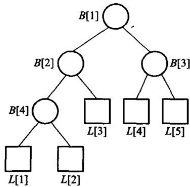
图 9.4 含有 5 个选手的赢家树
