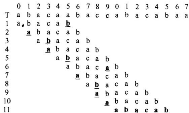
图 4.6 朴素匹配的示例
