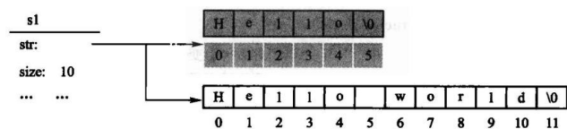
图 4.4 赋值运算示意图
