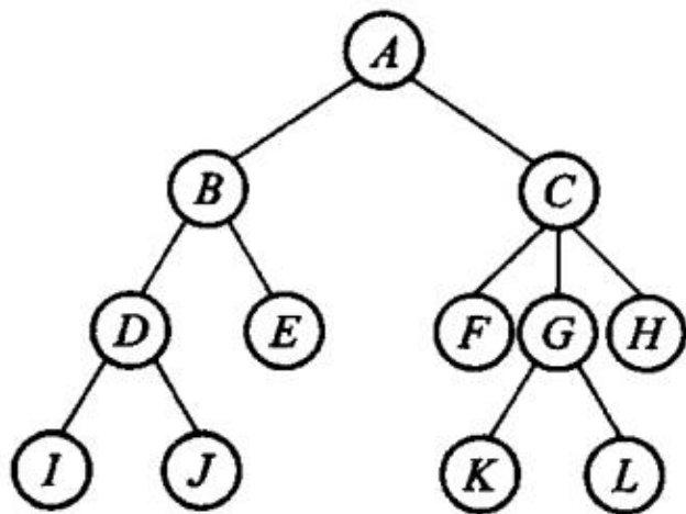
图 6.1 树形表示法
