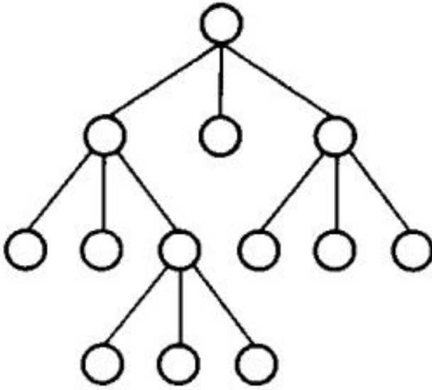
(a) 满 3 叉树
