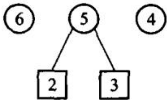
(b) 过程 2
