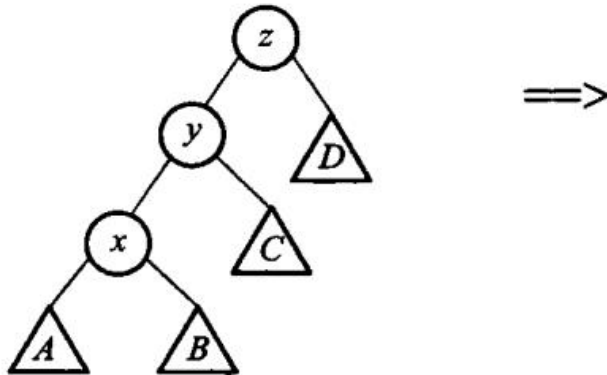
(a) 结点 x、结点 y、结点 z 为一字形的树结构
