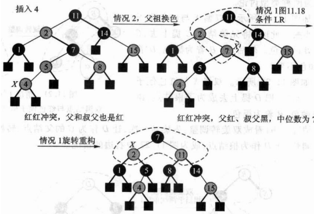
图 11.20 红黑树插入示例
