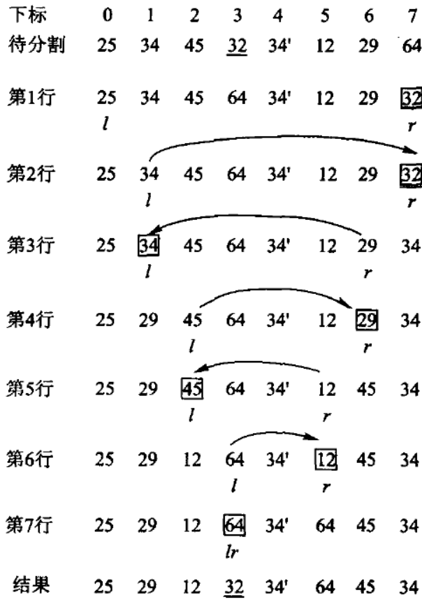
图 8.7 一趟分割的过程。分割是快排的全部工作量所在：它是 O(n) 的一次线性扫描，而分得均不均匀决定了递归有多深——每次都平分是 O(n \log n) ，每次只切下一个元素就退化成 O(n^2) 。
