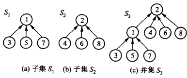
图 6.11 集合的父指针表示与并集：(a) 子集 S_1 、(b) 子集 S_2 各是一棵树，(c) 合并后 S_1 的根挂到了 S_2 的根下。
