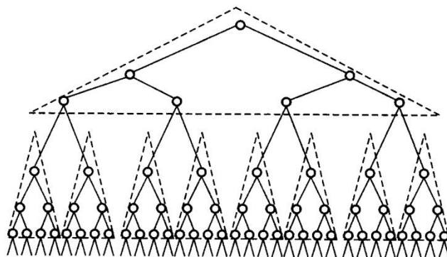
图 11.3 多分树
