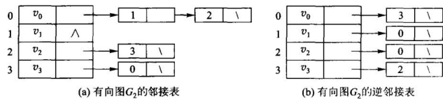
图 7.13 有向图 G_2 的邻接表和逆邻接表表示
