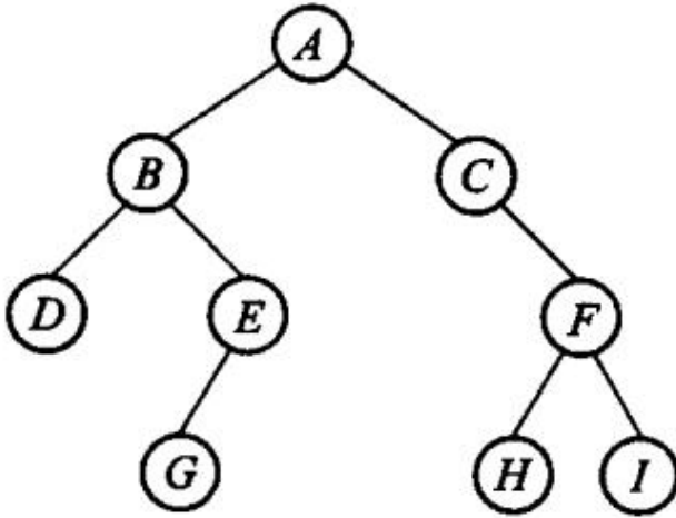
图 5.5 二叉树示例
