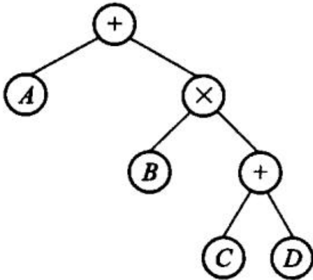
图 5.6 表达式树
