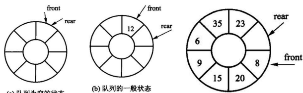
图 3.12 牺牲一格的循环队列（8 格数组最多放 7 个元素）：(a) 空，front == rear；(b) 一般状态；(c) 满， (rear + 1) \% (n + 1) == front 。
