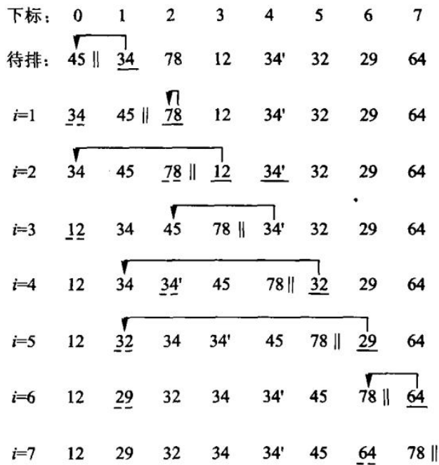
图 8.1 插入排序
