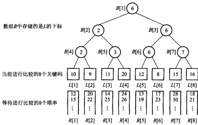
图 9.5 8 路归并的赢家树
