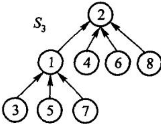
(c) 并集 S_3 ; 图 6.11 集合的表示方法
