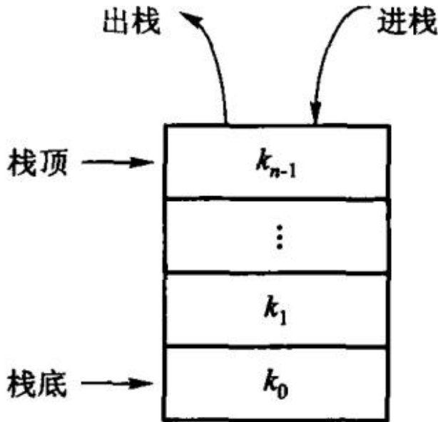
图 3.1 栈的示意图
