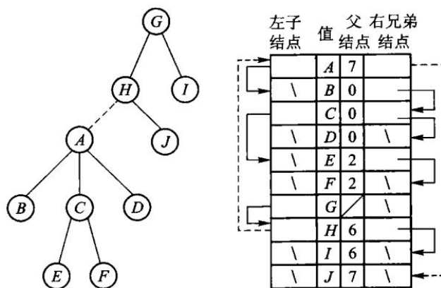
图 6.8 使用静态“左子/右兄”实现对树的归并
