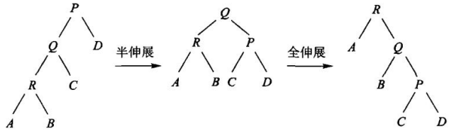
图 12.42 半伸展与全伸展的区别。
