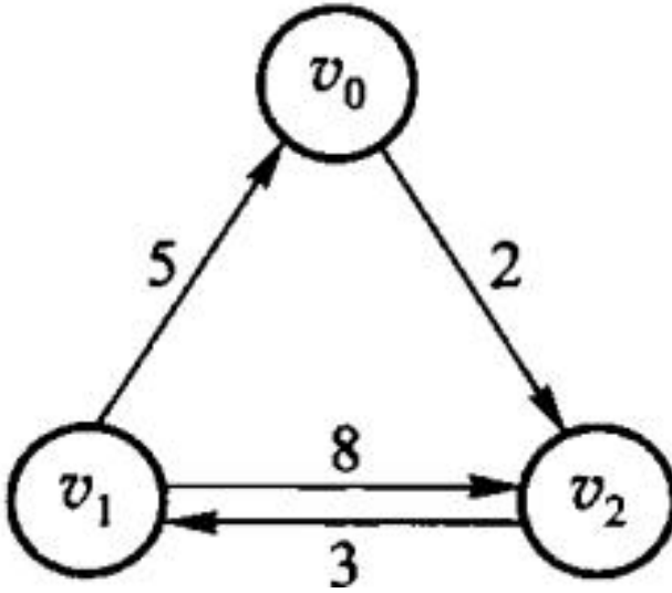
图 7.20 每对顶点间最短路径的示例。Floyd 从相邻矩阵 adj^{(0)} 出发，第 k 轮允许把 v_k 当中转点，得到 adj^{(k)} ； n 轮之后每一格就是最短路径长度（原书图 7.21 逐轮列出了这个迭代过程）。三重循环的次序不能换：中转点必须在最外层，否则 adj^{(k)} 还没算完就被拿去用了。
