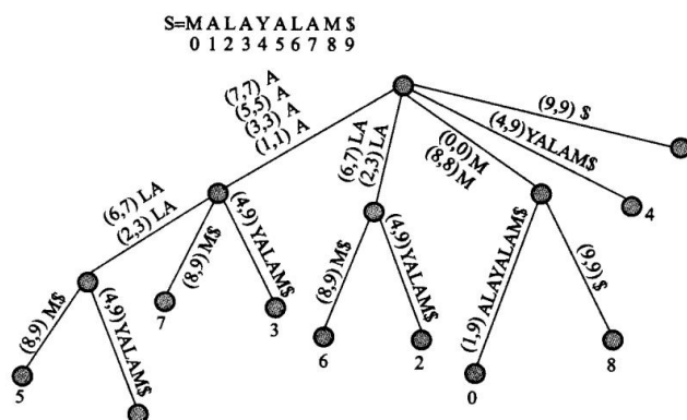
图 12.47 带路径压缩的后缀树
