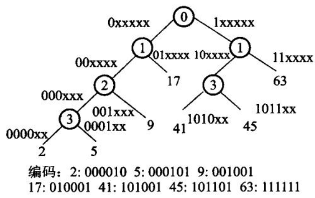
图 12.20 压缩后的 PATRICIA Trie。内部结点不再逐位下降，而是各自记住「该比第几位」。
