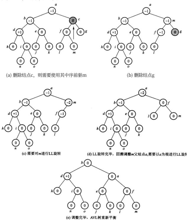
图 12.36 删除的例子：(a) 删有两个孩子的结点 c ，先用它的中序前驱 m 顶替，再删到叶那一层；(b) 删结点 g 之后 m 失衡；(c) 需要对 m 作 LL 旋转；(d) 转完 m 之
