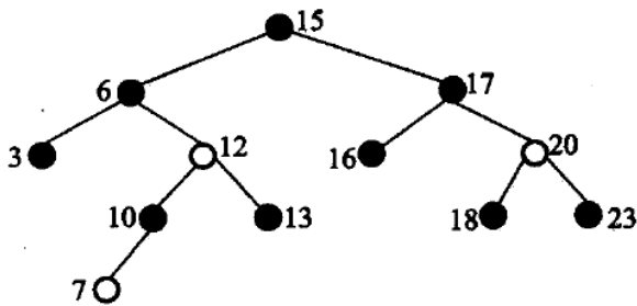
图 11.31 红黑树
