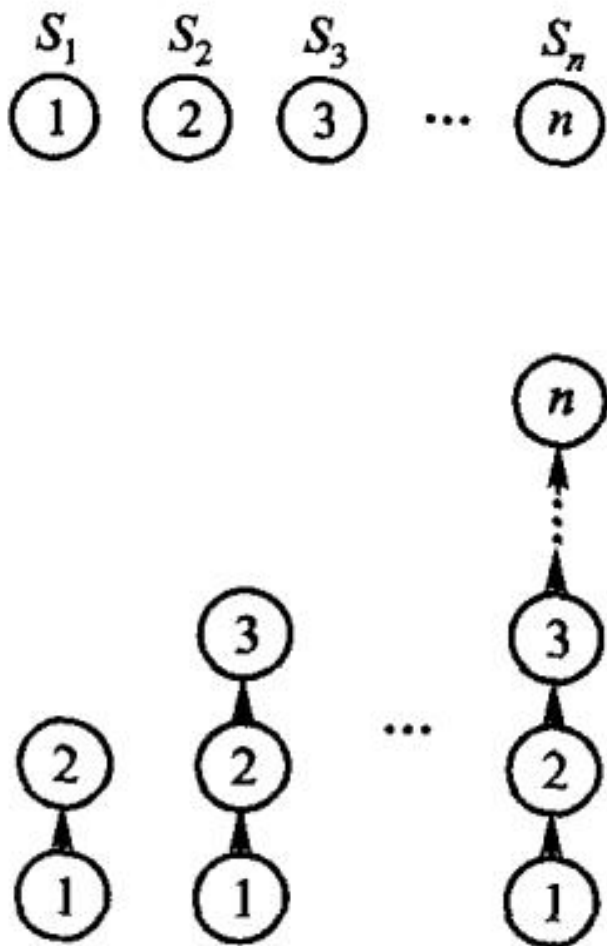
图 6.12 不采用重量权衡时，反复合并可能形成极端退化的树。
