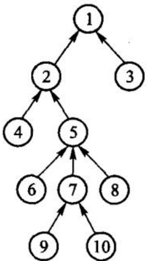
(a) 路径压缩之前
