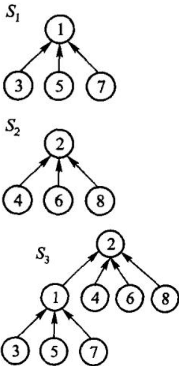
图 6.11 集合的父指针表示与并集。
