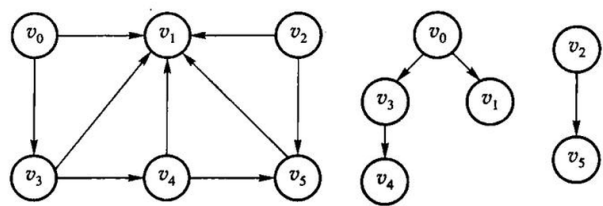
图 7.9 (a) 一个有向图；(b) 它的生成森林——两棵有向树，弧互不相交，顶点合起来是原图的全部顶点。
