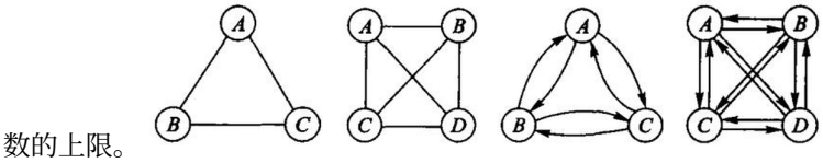
图 7.3 完全图: 左两幅是 3 个和 4 个顶点的 (a) 无向完全图, 右两幅是对应的 (b) 有向完全图。无向完全图每对顶点之间一条边, 有向完全图每对之间两条方向相反的弧。
