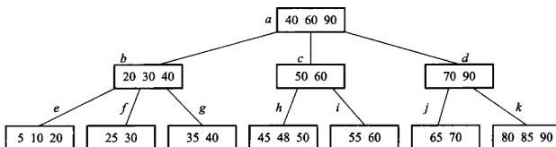
图 11.11 从图 11.9 的 3 阶 B+ 树里删掉 75 之后。内部结点上那份 75 的复写可
