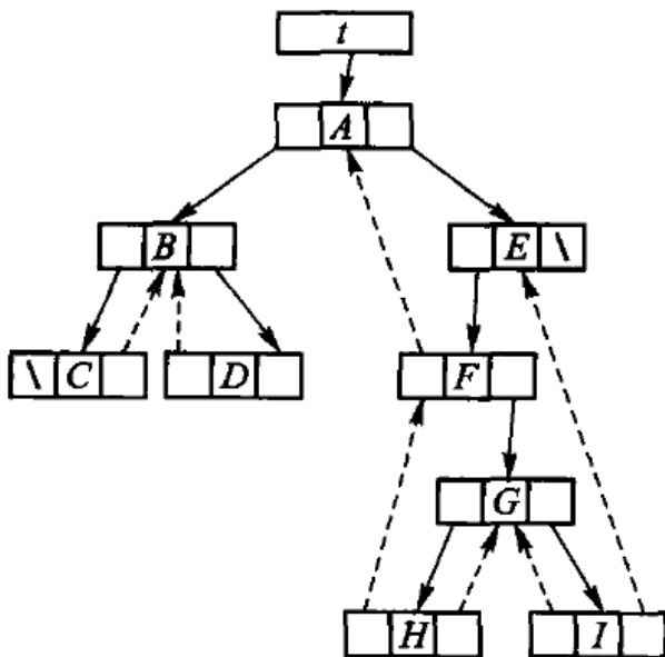
图 5.23 中序穿线（线索）二叉树。虚线是借空指针存下的中序前驱/后继，节点里另加一位标志区分「这根指针是孩子还是线索」。有了它，中序遍历不用栈也不用递归。
