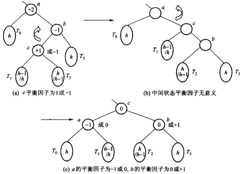
图 12.33 RL 型的双旋转，LR 型对称。中间那步的平衡因子没有意义（图中的 (b)）；转完之后 a 的因子是 -1 或 0 、 b 的因子是 0 或 +1 ，取决于被提上来的那
