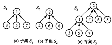
图 6.11 集合的父指针表示与并集: (a) 子集 S_1 、(b) 子集 S_2 各是一棵树, (c)
