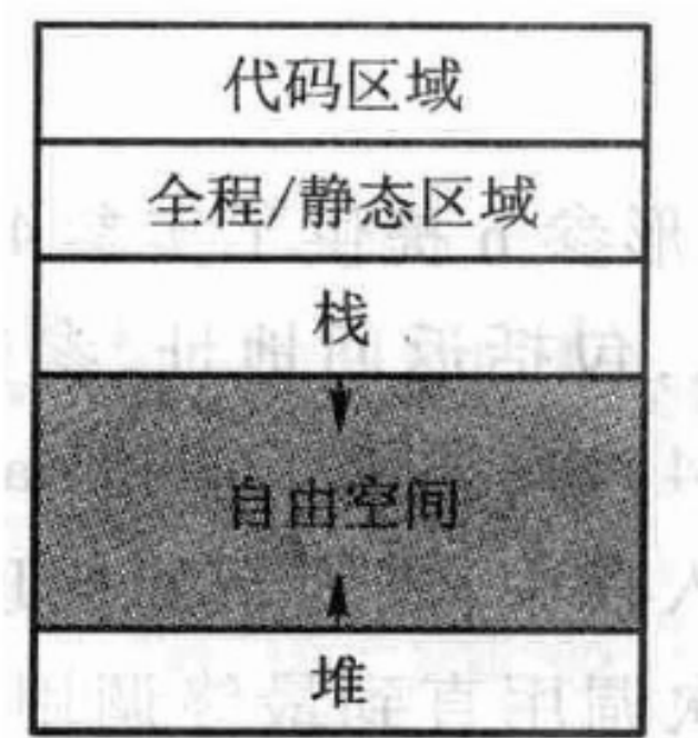
图 3.6 运行时存储器的组织形式：栈区放具有后进先出特征的数据（函数调用），堆区放不符合 LIFO 的动态分配（例如 new 出来的对象）。 栈区里一格一格压着的就是活动记录，它至少包含这些内容：
