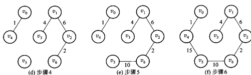
图 7.25 Kruskal 算法在同一张图 7.23 上的步骤（同样跨两页，(a)(b)(c) 与 (d)(e)(f) 各一张）。中间过程是一片森林，直到最后才连成一棵树；判断「这条边会不会成环」就是判断两个端点是不是已经在同一棵树里——这正是第 6 章并查集的用处。两个算法走的路不同，得到的总权相同。
