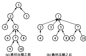
图 6.13 查找根结点时把沿途父指针直接改到根: (a) 是压缩之前的树, (b) 是对结点 7 调用一次 find 之后的样子——路径 7 \rightarrow 5 \rightarrow 2 上的结点都被直接改挂到根 1 下,而 9、10 仍留在 7 下面。
