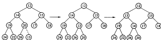
图 5.15 在图 5.14 的最小堆里插入 13：13 从末尾一路上浮，停在父结点比它小的地方。
