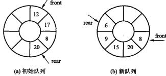
图 3.11 把数组看成环之后的样子：(a) 初始队列里有 12、17、8、20 四个元素；(b) 两次出队、三次入队之后，队列变成 8、20、15、9、6。入队增加 rear ，出队增加 front ，两者都在环上顺时针走。
