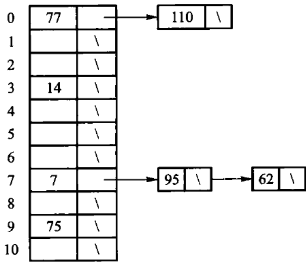
图 10.7 中每个表槽只是链头,同址键挂在同一条链上。原书这张图存 7 个数、散列表有 11 个槽、散列函数是 h(K) = K \bmod 11 ,插入顺序为 77、7、110、95、14、75、62: 结果有 2 个值散列到第 0 槽、1 个到第 3 槽、3 个到第 7 槽、1 个到第 9 槽。查找失败只需走完对应链,不看其他桶;删除也只摘掉链中结点。若每条链内部无序,成功查询平均看半条链,失败查询看整条链,这正是上面 ASL 公式中 \alpha/2 与 \alpha 的来源。
