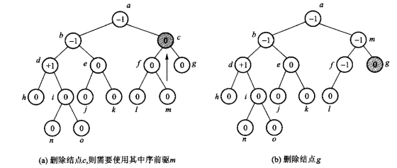
图 12.35 删除之后的调整。删除比插入麻烦：插入最多转一次就结束，删除可能一路向上每层都要转。
