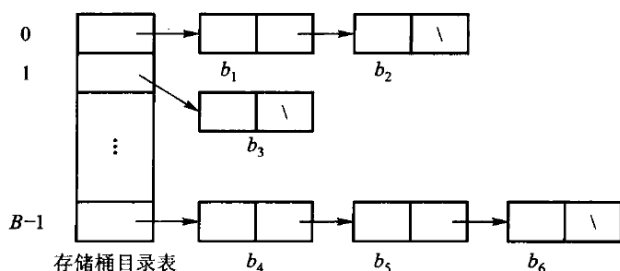
图 10.8 具有 B 个存储桶的散列文件组织。存储桶目录表存 B 个指针，各指向对应桶的第一个页块；1 号桶只有一个页块， B-1 号桶由 b_4 、 b_5 、 b_6 三块串成，每桶最后一块的指针为空。检索一次要一次访外读目录表、再逐块查桶，平均访外次数约为桶内页块数的一半——所以理想状态是每个桶只有一个页块，这也解释了为什么文件增长后需要重新组织、改散列函数并加长目录表。第 9 章和第 11 章讨论的正是这类「代价按访外次数计」的结构。
