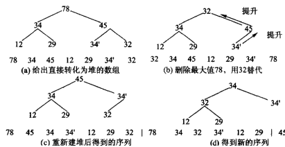
图 8.4 堆排序：(a) 待排序列建成最大堆；(b) 取走最大值 78，用末尾的 32 填上；(c) 重新筛选后又是一个堆；(d) 重复下去，每取一次就把一个最大值放到已排好的那一段。建堆是 O(n) (5.5.1a 证过)，此后 n-1 次筛选各 O(\log n) ，合计 O(n \log n) ——而且不需要额外数组。
