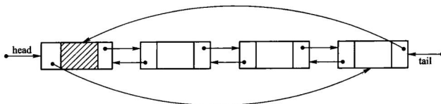
图 2.15 循环双链表示意图
