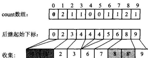
图 8.9 桶式排序示意图
