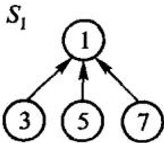
图 6.10 用每个结点的父指针表示树。
