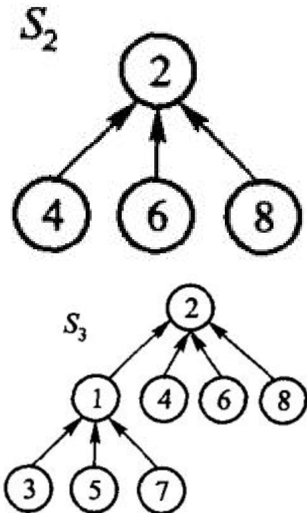
图 6.11 集合的父指针表示与并集。
