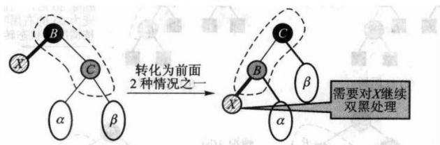
图 11.24 情况 3 双黑的兄弟结点为红色
