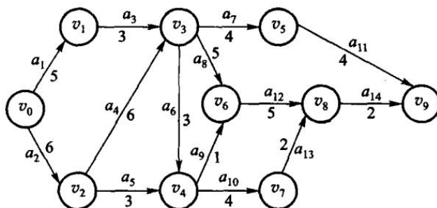
图 7.30 上机题 2 的图例
