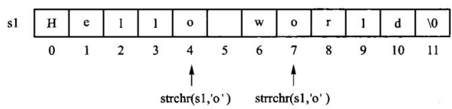
图 4.2 在字符串 s1 中寻找并定位给定字符 o' 的位置
