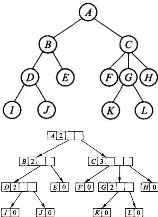
图 6.9 树的动态表示法。
