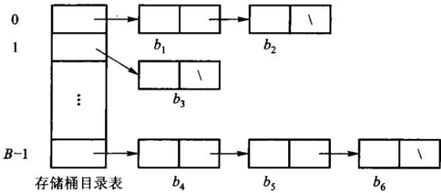
图 10.8 散列文件组织
