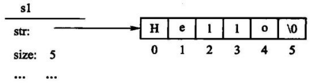
图 4.3 创建字符串的示意图
