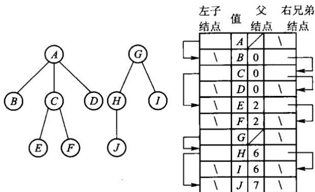
图 6.7 左孩子—右兄弟表示法把任意的树压成两个链接域。
