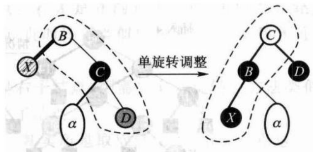
图 11.21 情况 1(a):
