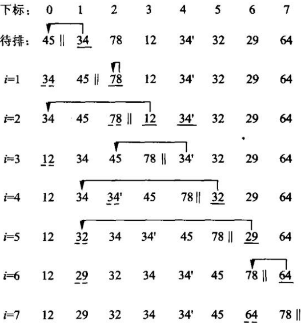
图 8.1 插入排序
