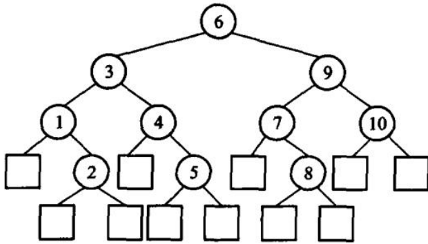
图 5.3 扩充二叉树
