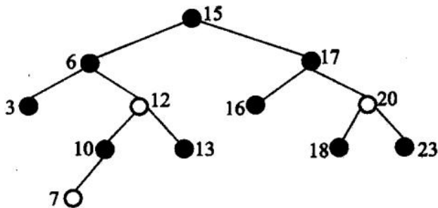
图 11.31 红黑树
