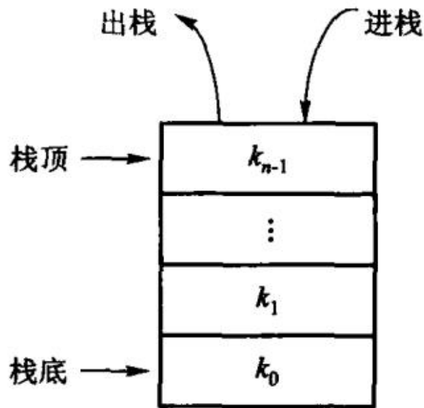
图 3.1 栈的示意图
