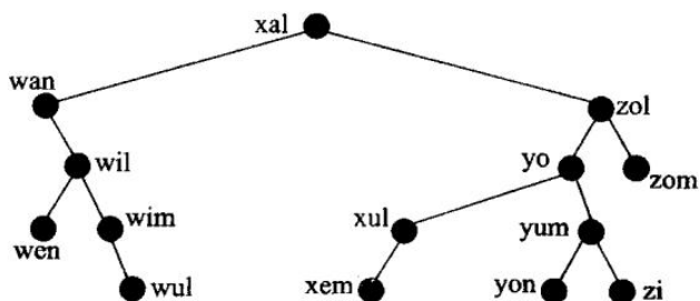
图 12.21 二叉搜索树
