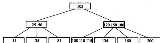
图 11.27 习题 9. 的 4 阶 B 树
