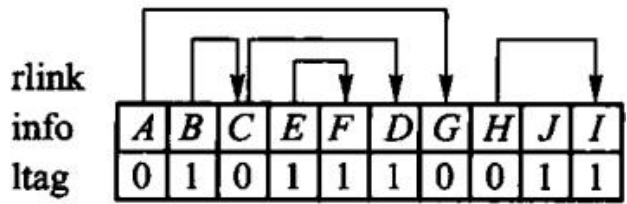
图 6.14 先根序列配合右链下标还原树形。
