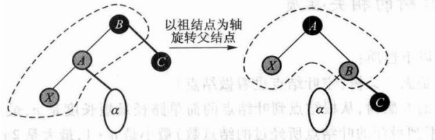
图 11.17 父结点是红色，叔父结点是黑色的情况，旋转解决红红冲突
