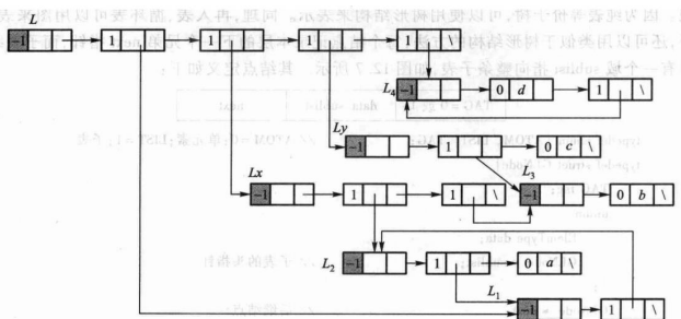
图 12.9 带表头结点的循环广义表
