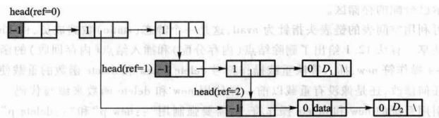
图 12.8 带头结点的广义表
