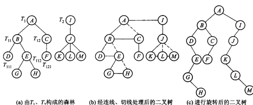
图 6.3 森林转换为二叉树
