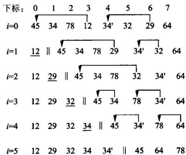
图 8.5 冒泡排序
