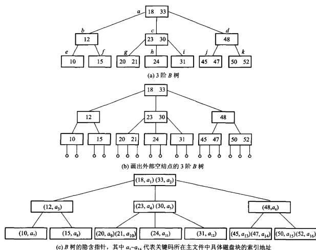
图 11.5 同一棵 3 阶 B 树的三种画法：(a) 通常的画法；(b) 把外部空结点画出来；(c) 画出隐含指针—— a_1 \sim a_{16} 是关键词在主文件里对应磁盘块的索引地址。 B 树 的关键词在内部结点上也带着数据地址，这正是它与后面 B+ 树的分水岭。
