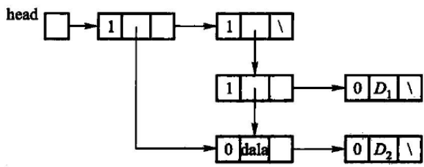
图 12.7 没有头结点的广义表。
