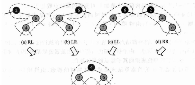
图 11.18 叔父为黑时一共四种种子结构 (LL、LR、RL、RR)。四种的实质是同一件事：取「双红结点 + 祖父」这三个键的中位数当新的子根、着黑，另外两个当它的孩子、着红。每个结点的阶（黑高）都不变，调整到此结束。
