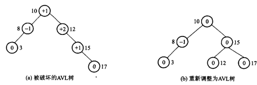
图 12.30 (a) 插入之后被破坏的 AVL 树；(b) 旋转之后重新变成 AVL 树。旋转只动局部几根指针，中序次序保持不变——这是所有平衡树旋转的共同前提。
