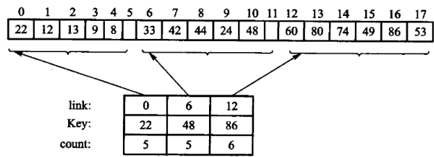
原书图 10.3 把主表分成三块：
