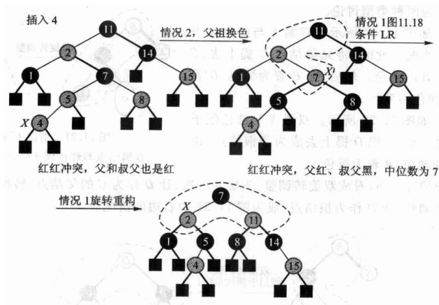
图 11.20 一次插入引发的红红冲突调整全过程。
