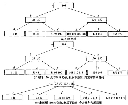
图 11.8 在一棵 (a) 5 阶 B 树上连续删除: (b) 删 120——先与中序后继交换再删，删后下溢，向左邻借一个关键码; (c) 接着删 150——同样先交换，删后下溢而两侧都借不到，只能合并，合并又让父结点下溢，一路传到根。
