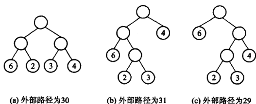
图 5.18 三棵外部结点权值同为 6、2、3、4 的扩充二叉树。(a) 6 \times 2 + 2 \times 2 + 3 \times 2 + 4 \times 2 = 30 ; (b) 6 \times 2 + 2 \times 3 + 3 \times 3 + 4 \times 1 = 31 ; (c) 6 \times 1 + 2 \times 3 + 3 \times 3 + 4 \times 2 = 29 。(c) 最小，它就是这组权值的 Huffman 树——权越大的叶离根越近，总长就越小。
