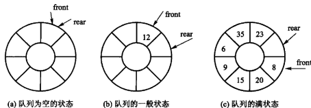
图 3.12 牺牲一格的循环队列（8 格数组最多放 7 个元素）：(a) 空， front == rear ；(b) 一般状态；(c) 满， (rear + 1) \% (n + 1) == front 。
