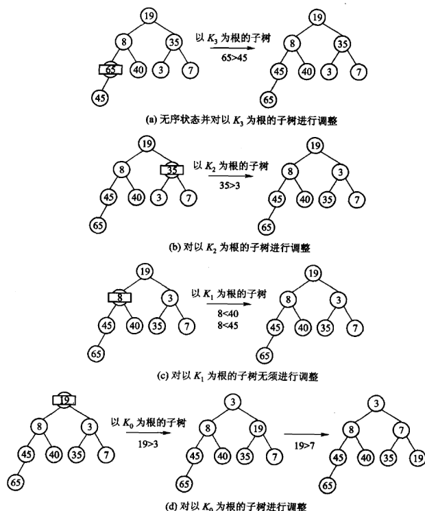
图 5.17 建堆过程示例（原书图 5.17 的筛选法）。倒着做的理由是：对某个结点下沉时，它的两棵子树必须已经是堆——从最后一个非叶结点往前扫，正好保证这一点。叶结点本身就是堆，所以后半结点一次都不用碰。
