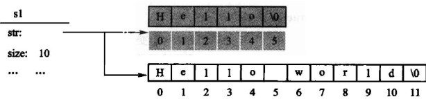
图 4.4 赋值运算： String 按当前串长动态调整空间，这就是「变长管理」的全部含义。注意图上那块灰色的旧空间——它必须释放，而且必须在新空间准备好之后再释放。原书正文说到了这一步，却没有给出拷贝赋值的代码；漏掉它， String b = a; 就是二次释放。
