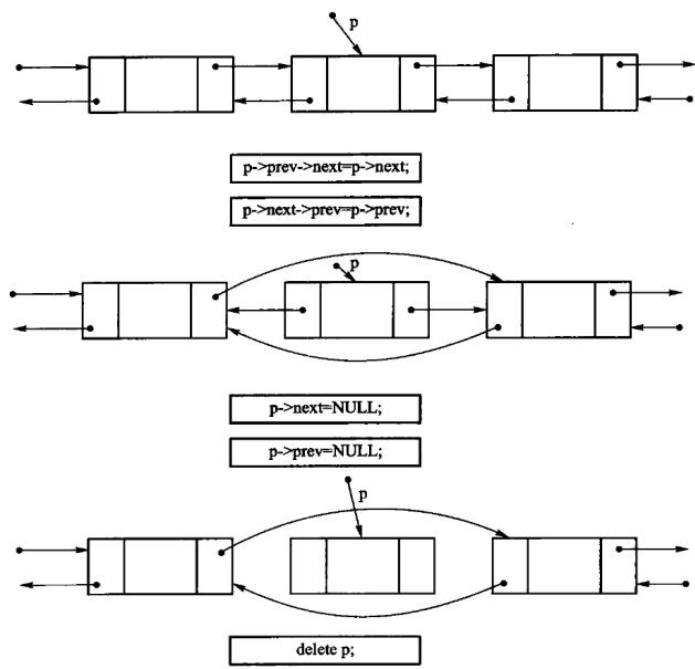
图 2.11 双链表的删除操作示意。摘链之后把 p 自己的两根指针置空再释放，是为了让「已删除的结点还被别人拿着」这种错误尽早暴露。 在 p 之后插入新结点 q ，先让 q 认好左右邻居，再让邻居认 q ： text original-listing=" 原书 2.3.2 节插入双链结点的指针操作，作为原书记录 原样引用" q->prev = p; q->next = p->next; p->next = q; q->next->prev = q;
