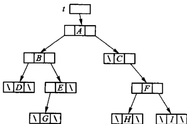
图 5.8 图 5.5 那棵树的二叉链表存储结构。数一数图里的空指针： n 个结点的二叉链表恰有 n + 1 个空链域（5.1.3 的性质 5），线索二叉树就是要把它们利用起来。
