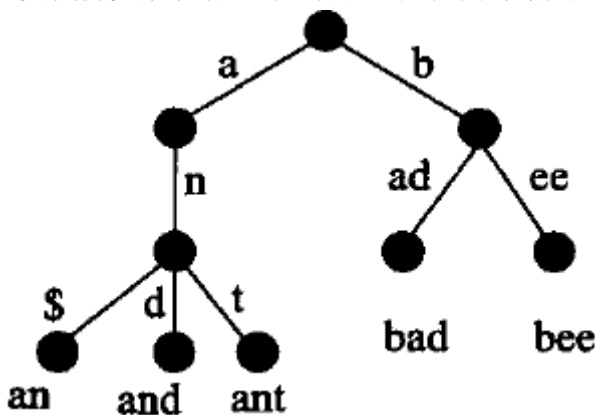
图 12.18 对 Trie 树的改进: 只保存实际用到的分支, 代价是查一层要在表
