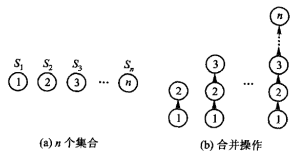
图 6.12 不采用重量权衡时，反复合并可能形成极端退化的树：(a) 起初是 n 个单元素集合，(b) 每次都把大树挂到小树下，最后退化成一个长链。
