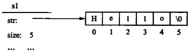
图 4.3 创建字符串：对象里只有一个指针和一个长度，字符本体在堆上。 再写 String s2 = "Hello world"; s1 = s2; ，新内容比旧的长，装不下，于是必须先另开一块新数组、把内容复制过去，旧数组（图 4.4 中的灰格）释放掉， str 改指新数组：
