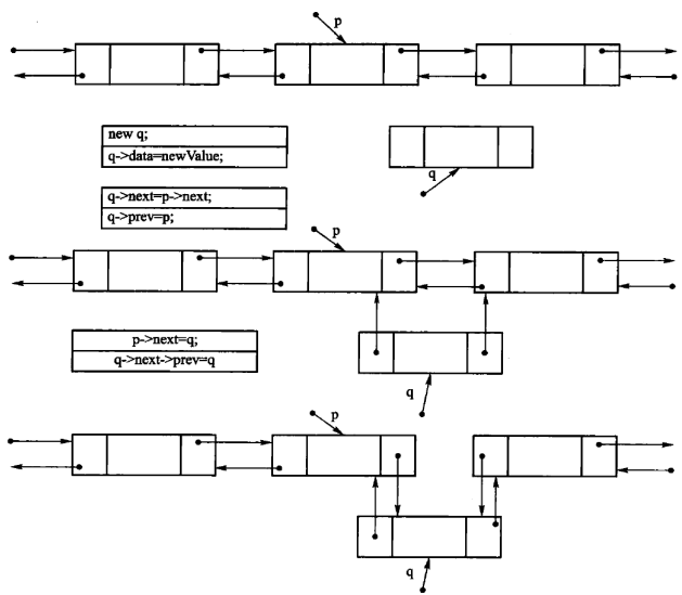
图 2.12 双链表插入操作示意。四条赋值的次序可以变，但「先让新结点指向两侧、再改两侧指向新结点」这个方向不能反——否则改到一半就丢了原来的
