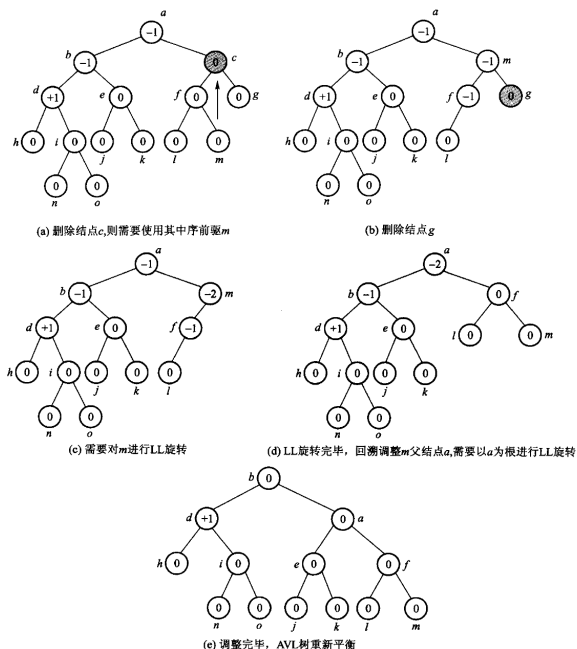
图 12.36 删除的例子（原书跨两页，(a)(b) 一页、(c)(d)(e) 一页）：(a) 删有两个孩子的结点 c ，先用它的中序前驱 m 顶替，再删到叶那一层；(b) 删结点 g 之后 m 失衡；(c) 需要对 m 作 LL 旋转；(d) 转完 m 之后回溯，父结点 a 又失衡，再以 a 为根作一次 LL 旋转；(e) 调整完毕，整棵树重新平衡。一次删除可能引发从被删结点一路到根的多次旋转，这是它与插入最大的不同。
