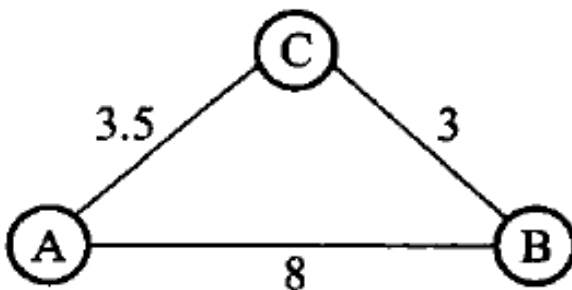
图 7.18 最短路径的示例：从 A 到 B 的最短路径是 A → C → B，并不是边数
