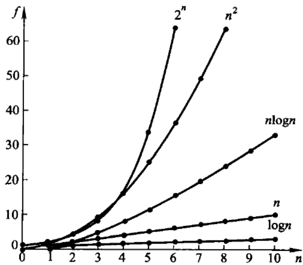
图 1.5 常用函数的增长趋势。 同一组 n 用数字排出来是这样：
