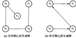
图 7.7 图 7.2 中 (a) 无向图 G_1 和 (b) 有向图 G_2 的一棵生成树。生成树上再加一条边必成环；边数少于 n - 1 则必不连通。
