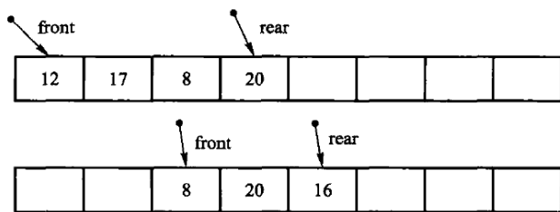
图 3.10 顺序队列的实现示意。出队让 front 后移，入队让 rear 后移；元素本身一个都不搬。
