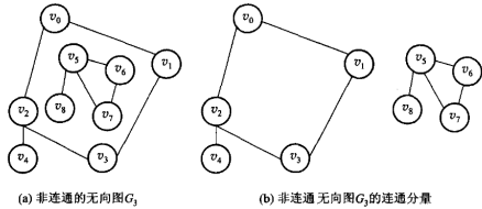
图 7.5 (a) 非连通的无向图 G_3 ；(b) G_3 的两个连通分量。「极大」是指再添任何一个顶点，子图就不连通了。
