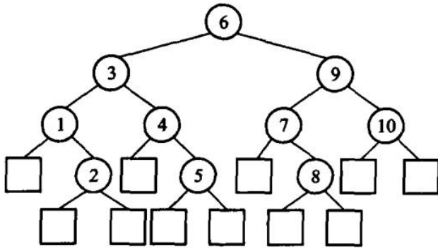
图 5.3 扩充二叉树
