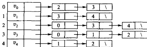
图 7.12 无向图 G_1 的邻接表表示。顶点数组的每一项挂一条链，链上是它的邻接点。无向图里一条边出现两次（ (u, v) 在 u 的表里，也在 v 的表里），所以边表结点共 2e 个。
