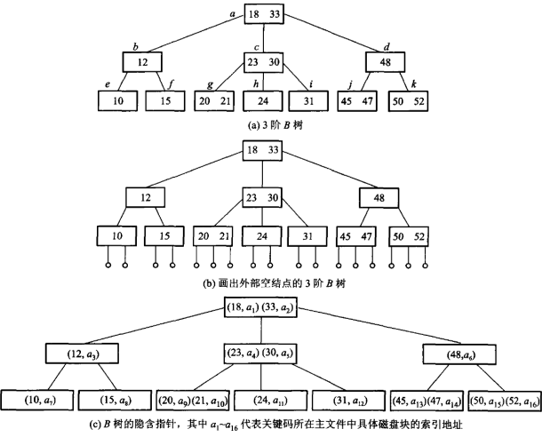
图 11.5 同一棵 3 阶 B 树的三种画法：(a) 通常的画法；(b) 把外部空结点画出来；(c) 画出隐含指针—— a_1 \sim a_{16} 是关键码在主文件里对应磁盘块的索引地址。 B 树的关键码在内部结点上带着数据地址，这正是它与后面 B+ 树的分水岭。
