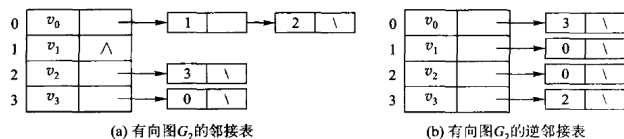
图 7.13 有向图 G_2 的 (a) 邻接表与 (b) 逆邻接表。逆邻接表里 v_i 的边表长度就是它的入度——7.4.3 节拓扑排序要的正入度。
