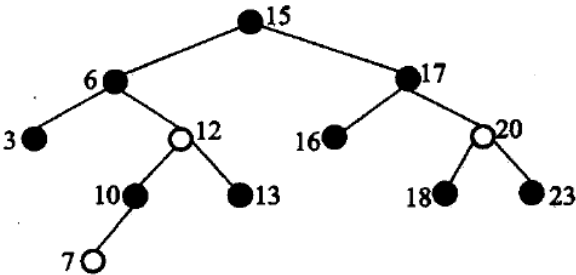
图 11.31 红黑树
