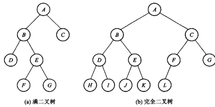
图 5.2 (a) 满二叉树；(b) 完全二叉树。
