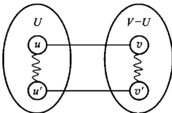
图 7.22 含 (u, v) 的回路。删掉 (u', v') 就消掉了回路，得到另一棵生成树 T' ；因
