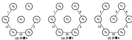
图 7.24 Prim 算法在图 7.23 上的六个步骤 (原书印在相邻两页上, (a)(b)(c) 一页、(d)(e)(f) 一页, 这里照原样分作两张)。注意每一步长出来的都是一棵连着的树——这正是它与 Kruskal 的区别。
