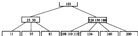
图 11.27 习题 9 的 4 阶 B 树
