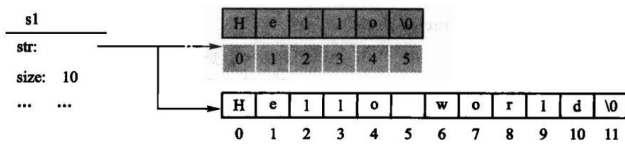
图 4.4 赋值运算示意图
