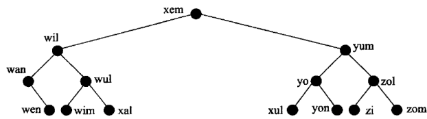
图 12.24 等权时的最佳二叉搜索树——形状尽量平衡。
