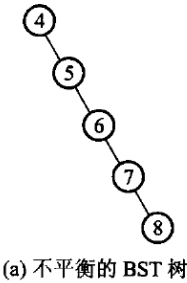
图 12.15 同一批关键码，形状可以从「接近完全二叉树」一直退化到「一条链」——检索代价随之从 O(\log n) 变成 O(n) 。
