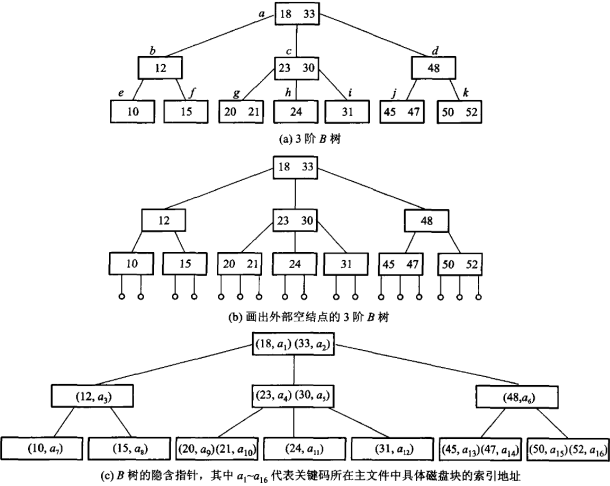
图 11.5 同一棵 3 阶 B 树的三种画法：(a) 通常的画法；(b) 把外部空结点画出来；(c) 画出隐含指针—— a_1 \sim a_{16} 是关键码在主文件里对应磁盘块的索引地址。 B 树的关键码在内部结点上也带着数据地址，这正是它与后面 B+ 树的分水岭。
