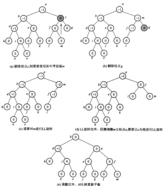
图 12.36 删除的例子 (原书跨两页, (a)(b) 一页、(c)(d)(e) 一页): (a) 删有两个孩子的结点 c, 先用它的中序前驱 m 顶替, 再删到叶那一层; (b) 删结点 g 之后 m 失衡; (c) 需要对 m 作 LL 旋转; (d) 转完 m 之后回溯, 父结点 a 又失衡, 再以 a 为根作一次 LL 旋转; (e) 调整完毕, 整棵树重新平衡。一次删除可能引发从被删结点一路到根的多次旋转, 这是它与插入最大的不同。
