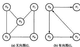
图 7.2 图的示例: (a) 无向图 G_1 , (b) 有向图 G_2 。本章后面反复拿这两张图举例。
