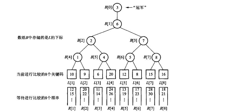
图 9.7 中内部结点保存败者，冠军另放在根外的槽位。替换冠军之后，新值只与路径上留下的败者依次比较。
