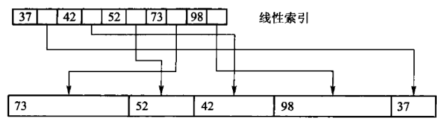
图 1.4 索引示例
