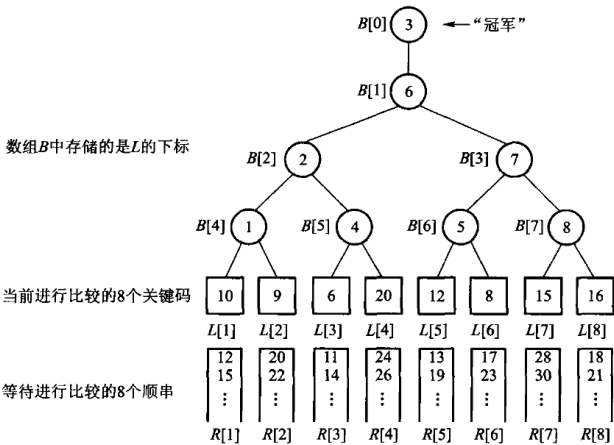
图 9.7 中内部结点保存败者，冠军另放在根外的槽位 B[0] 。方形外部结点 L[1..8] 是各路当前参与比较的关键码 10 9 6 20 12 8 15 16， B[0] = 3 指示最小关键码 6 在第三个顺串。替换冠军之后，新值只与路径上留下的败者依次比较。
