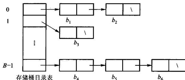
图 10.8 具有 B 个存储桶的散列文件组织。存储桶目录表存 B 个指针，各指向对应桶的第一个页块；1 号桶只有一个页块， B - 1 号桶由 b_4 、 b_5 、 b_6 三块串成，每桶最后一块的指针为空。检索一次要一次访外读目录表、再逐块查桶，平均访外次数约为桶内页块数的一半——所以理想状态是每个桶只有一个页块，这也解释了为什么文件增长后需要重新组织、改散列函数并加长目录表。第 9 章和第 11 章讨论的正是这类「代价按访外次数计」的结构。
