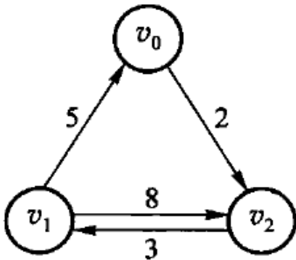
图 7.20 每对顶点间最短路径的示例。Floyd 从相邻矩阵 adj^{(0)} 出发, 第 k 轮新允许把 v_{k-1} 当中转点(代码里的 via 从 0 数起, 即 via = k-1 ), 得到 adj^{(k)} ; n 轮之后每一格就是最短路径长度 (逐轮结果见下面的图 7.21)。三重循环的次序不能换: 中转点必须在最外层 , 否则 adj^{(k)} 还没算完就被拿去用了。
