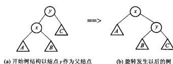
图 12.38 只有当被展开的结点已经是根的孩子时，才做单旋转：左边是旋转前，右边是旋转后。
