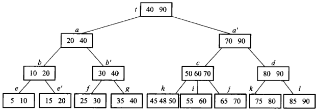
图 11.10 原书的例子：在图 11.9 的 3 阶 B+ 树中插入 15。沿 a 、 b 、 e 找到叶 e ，(5,10,15,20) 上溢，分裂为 e (5,10) 与 e' (15,20)，左结点的新最大码 10 复写到 b ； b 变成 (10,20,30,40) 再分裂为 b 与 b' ，20 复写到 a ； a 变成 (20,40,70,90) 又分裂为 a 与 a' ，两者的最大码 40、90 组成新根 t ，树增高一层。共读盘 3 次 ( a, b, e )、写盘 7 次 ( e, e', b, b', a, a', t )。原书采用的是「最大关键码复写」，所以与上面「最小关键码复写」的推演形状不同，道理相同。
