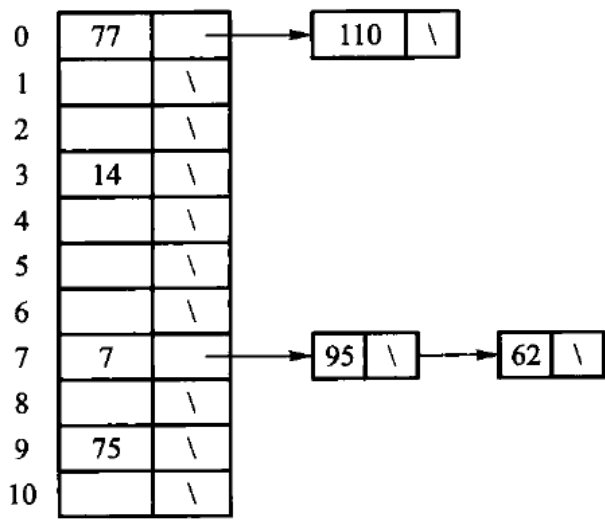
图 10.7 中每个表槽只是链头, 同址键挂在同一条链上。原书这张图存 7 个数、散列表有 11 个槽、散列函数是 h(K) = K \bmod 11 , 插入顺序为 77、7、110、95、14、75、62: 结果有 2 个值散列到第 0 槽、1 个到第 3 槽、3 个到第 7 槽、1 个到第 9 槽。查找失败只需走完对应链, 不看其他桶; 删除也只摘掉链中结点。若每条链内部无序, 成功查询平均看半条链, 失败查询看整条链, 这正是上面成功检索约 1 + \alpha/2 、以及 10.3.5 节表中不成功检索约 \alpha + e^{-\alpha} (主项是整条链长 \alpha ) 的来源。
