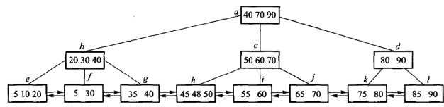
图 11.9 原书的 3 阶 B+ 树，采用「最大关键码复写」：上层每个关键码是对应子结点的最大关键码。扫描件中叶结点 f 印作 5 30，应为 25 30（父结点 b 的分界码是 20、30， f 里的键必须大于 20；图 11.10、11.11 中同一叶也都是 25 30）。
