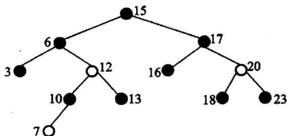
图 11.31 红黑树
