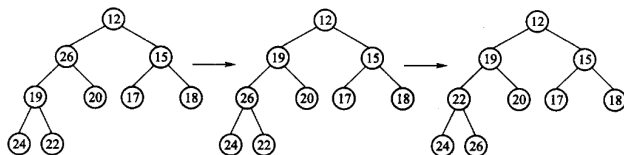
图 5.16 在图 5.14 的最小堆里删除 14: 末端元素填进空出来的位置, 再与较小的那个孩子逐层交换下沉, 直到它不大于自己的孩子。具体是: 14 在下标 1, 末端的 26 填进来; 它的孩子 19、20 里小的是 19, 26 > 19 , 交换; 再看孩子 24、22, 小的是 22, 26 > 22 , 交换; 26 到了叶子, 停。数组变成 12 19 15 22 20 17 18 24 26。
