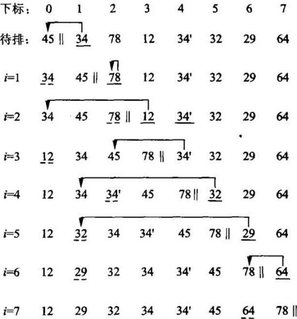
图 8.1 插入排序
