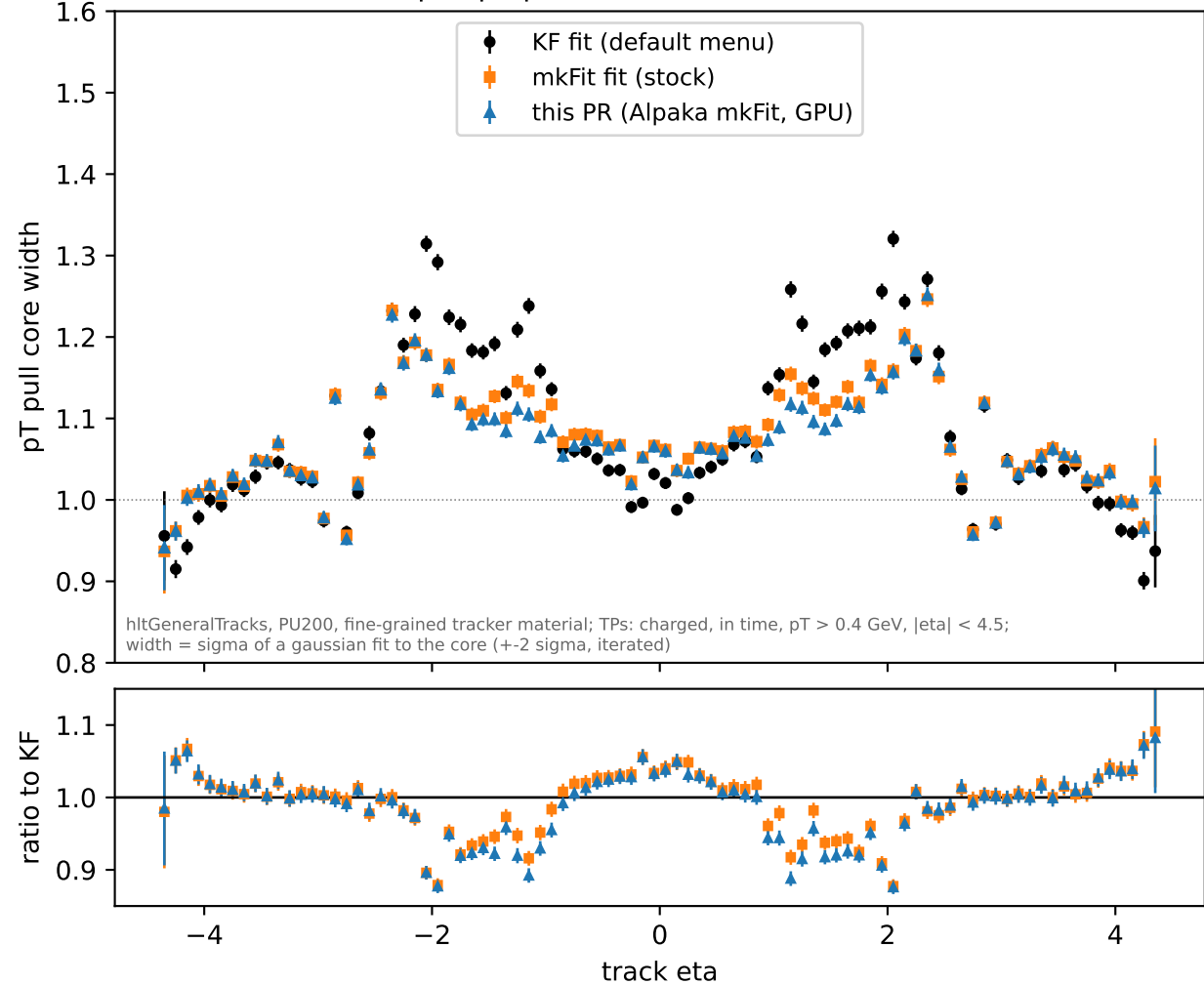
qcd: pT pull core width vs track eta
