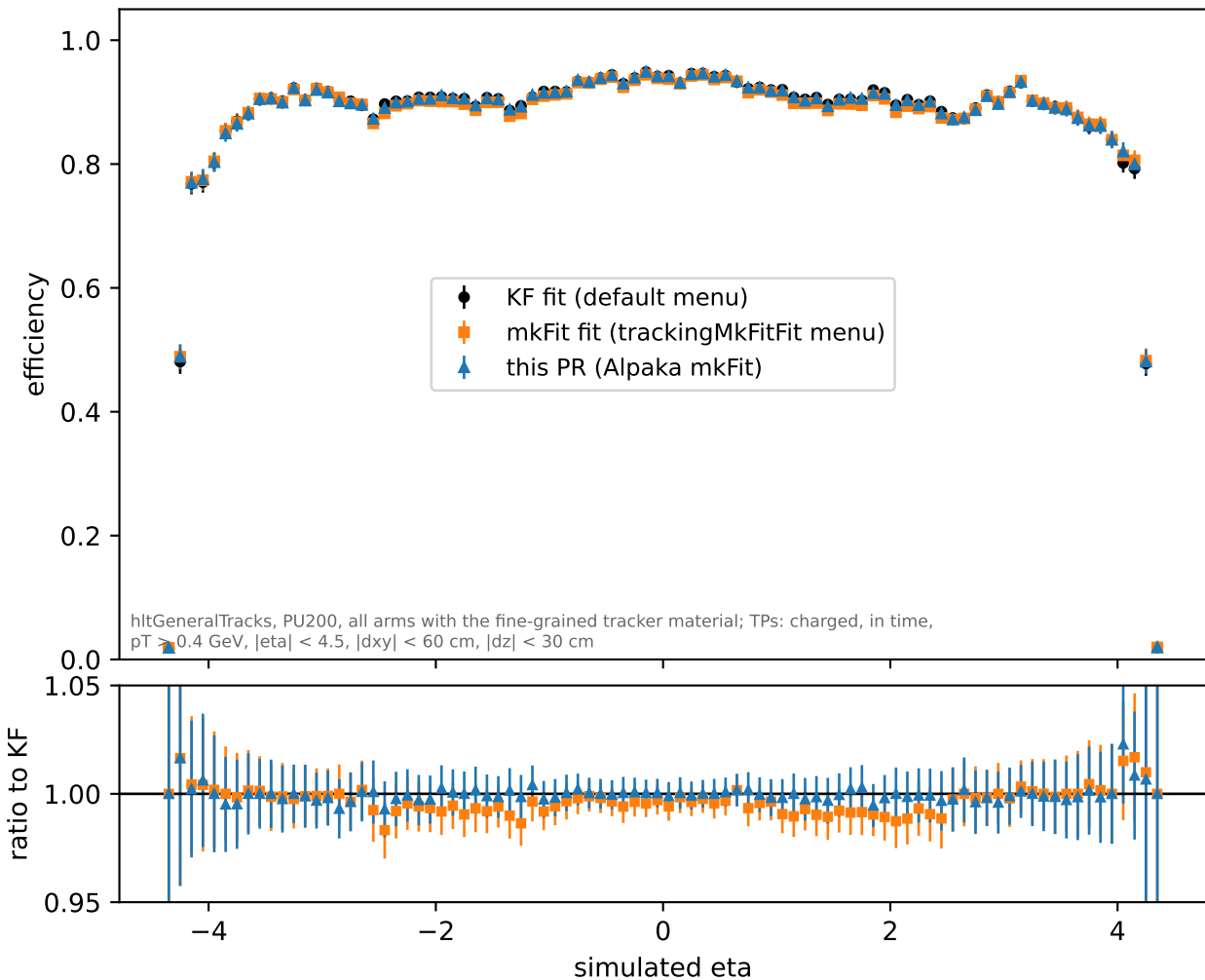
ttbar: efficiency vs simulated eta
