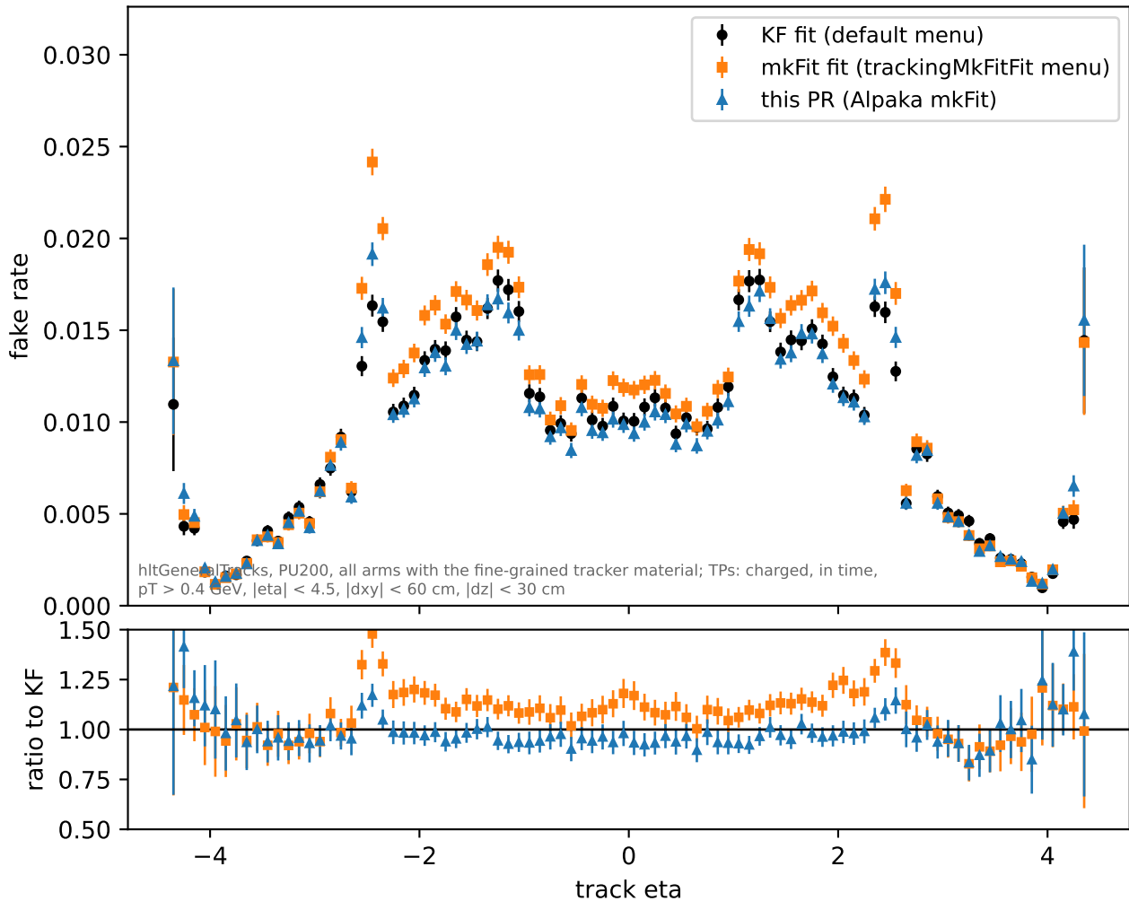
ttbar: fake rate vs track eta
