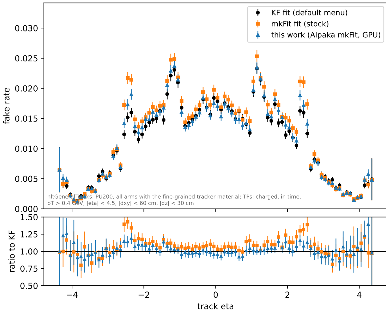
qcd: fake rate vs track eta
