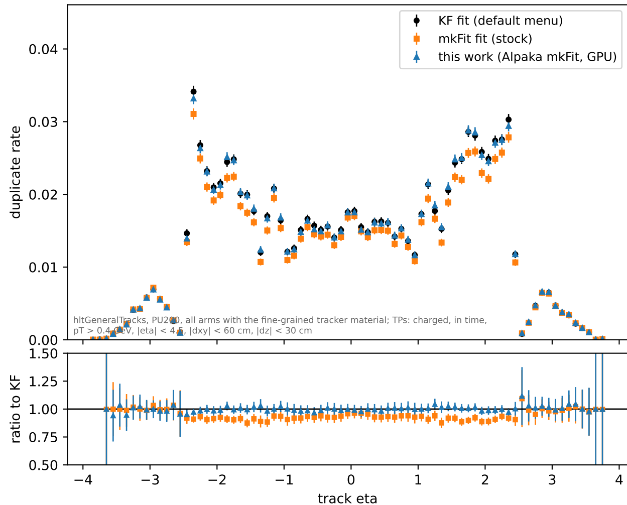
ttbar: duplicate rate vs track eta
