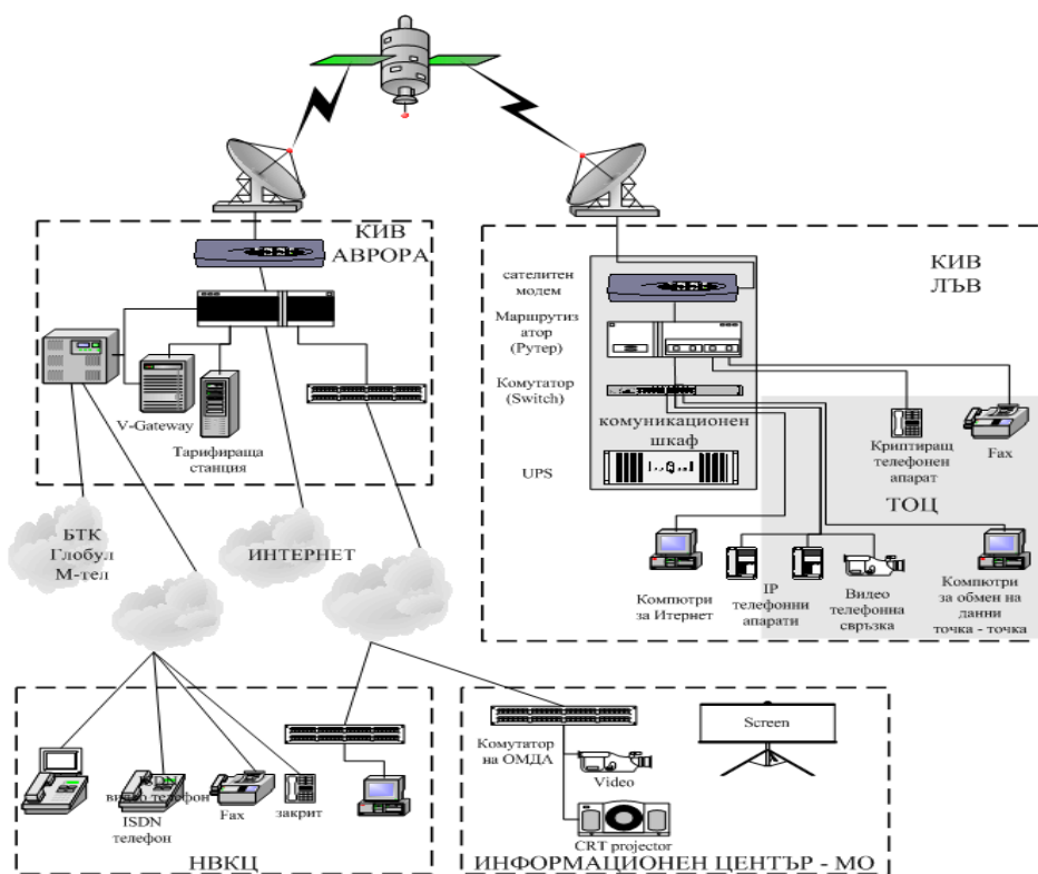
Фиг. 20. Спътникова система VSAT
