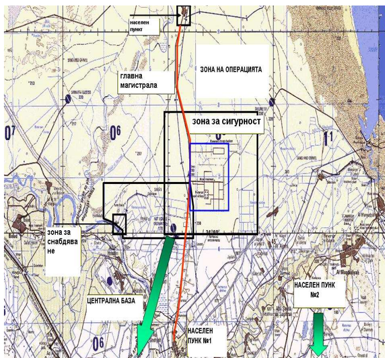
Фиг. 21. Схема на зоната за сигурност на оперативна база
