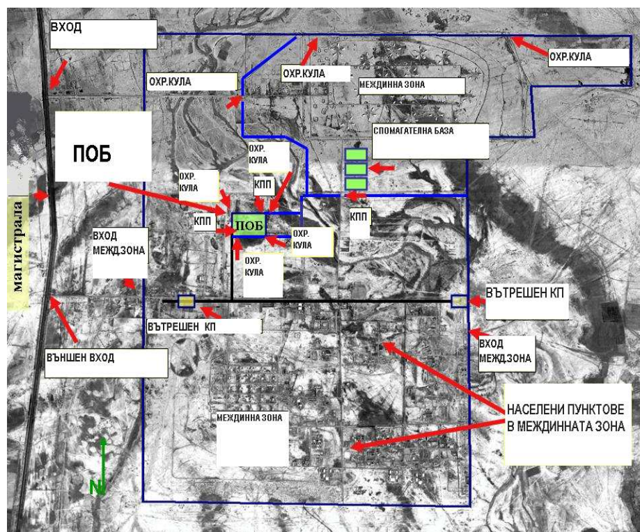
Фиг. 22. Схема на зоната за физическа сигурност на оперативна база
