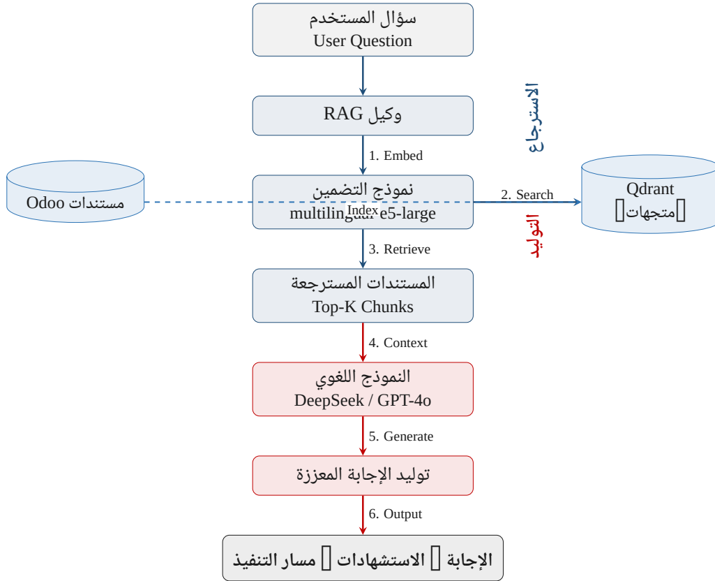
شكل 2-1: مخطط تدفق تقنية RAG في نظام بيان.
