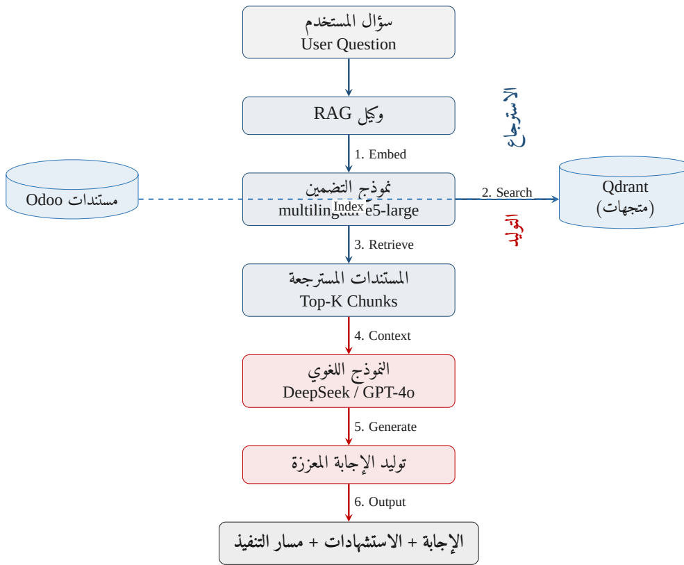
شكل 1-2: مخطط تدفق تقنية RAG في نظام بيان.
