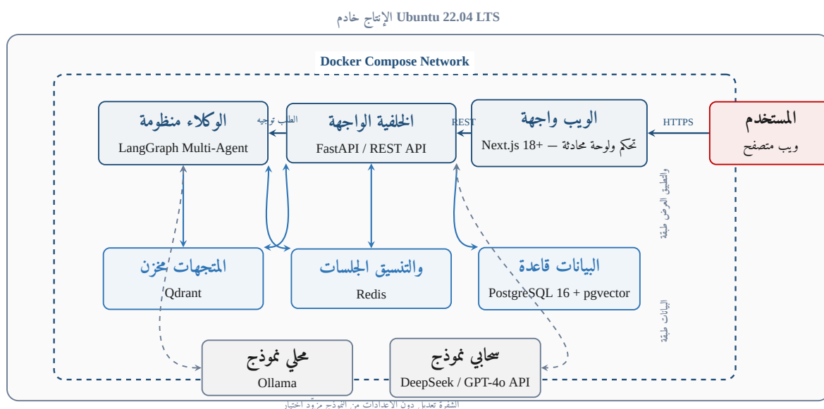
شكل 3-4: معمارية نشر نظام «بيان» عبر Docker Compose.
