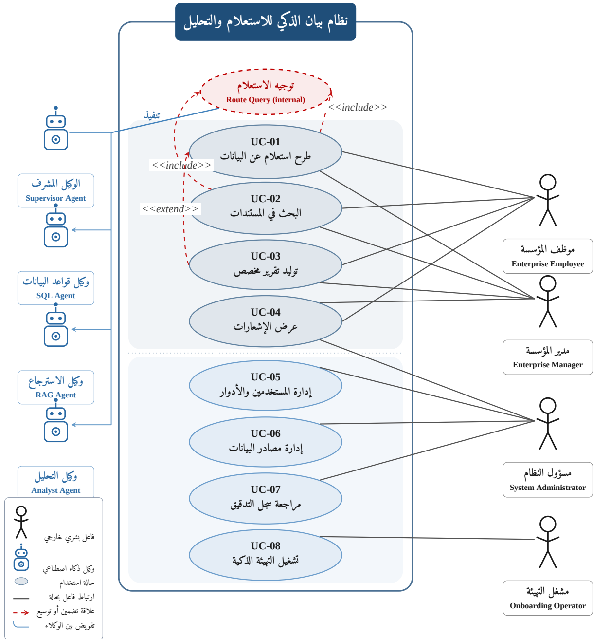
شكل 3-6: مخطط حالات الاستخدام لنظام «بيان» يُظهر تفاعل الفاعلين البشريين والوكلاء الآليين مع الحالات الثماني.
