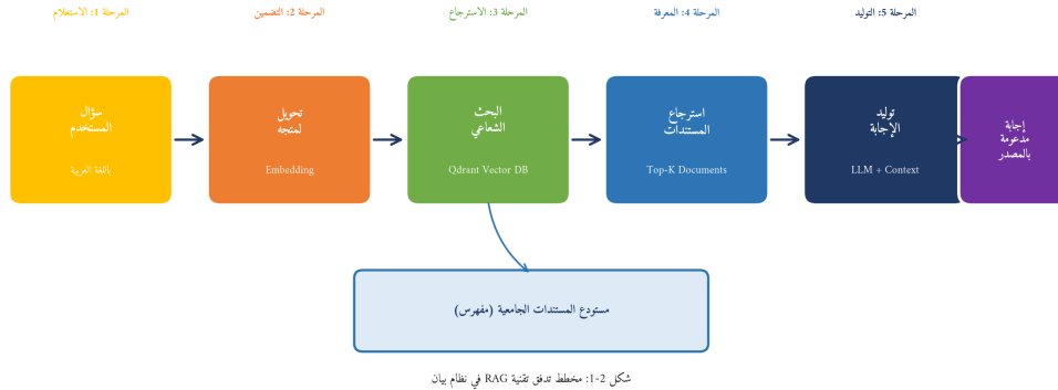
شكل 1-2: مخطط تدفق تقنية RAG في نظام بيان.
