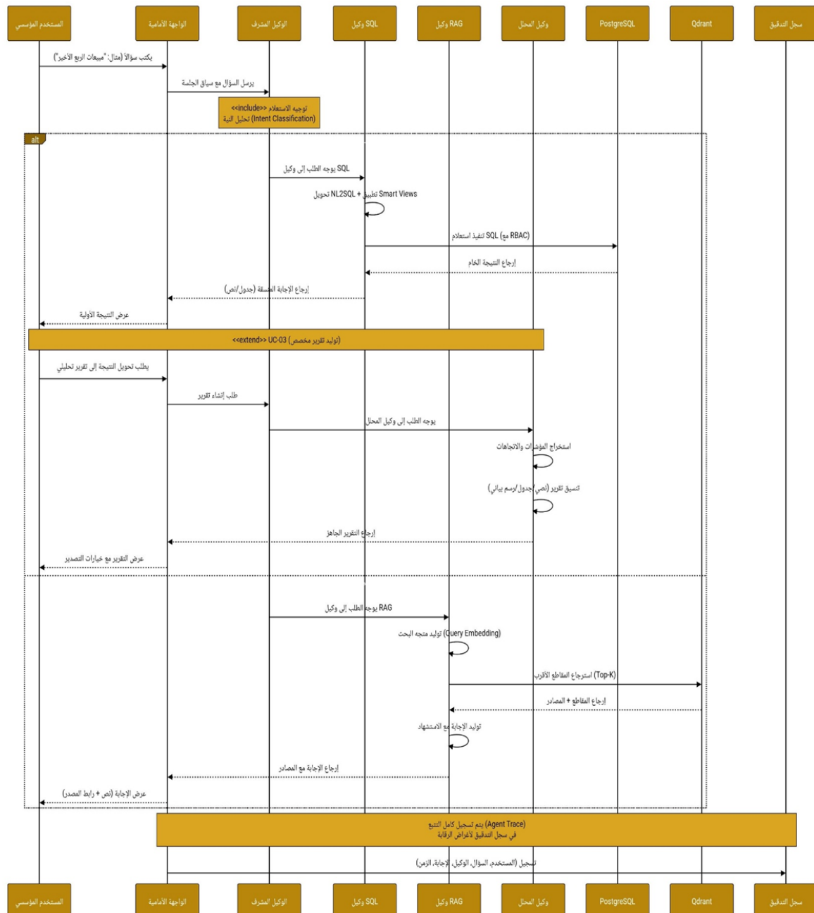
شكل 3-7: مخطط التسلسل لتدفقات الاستعلام والبحث وتوليد التقرير.
