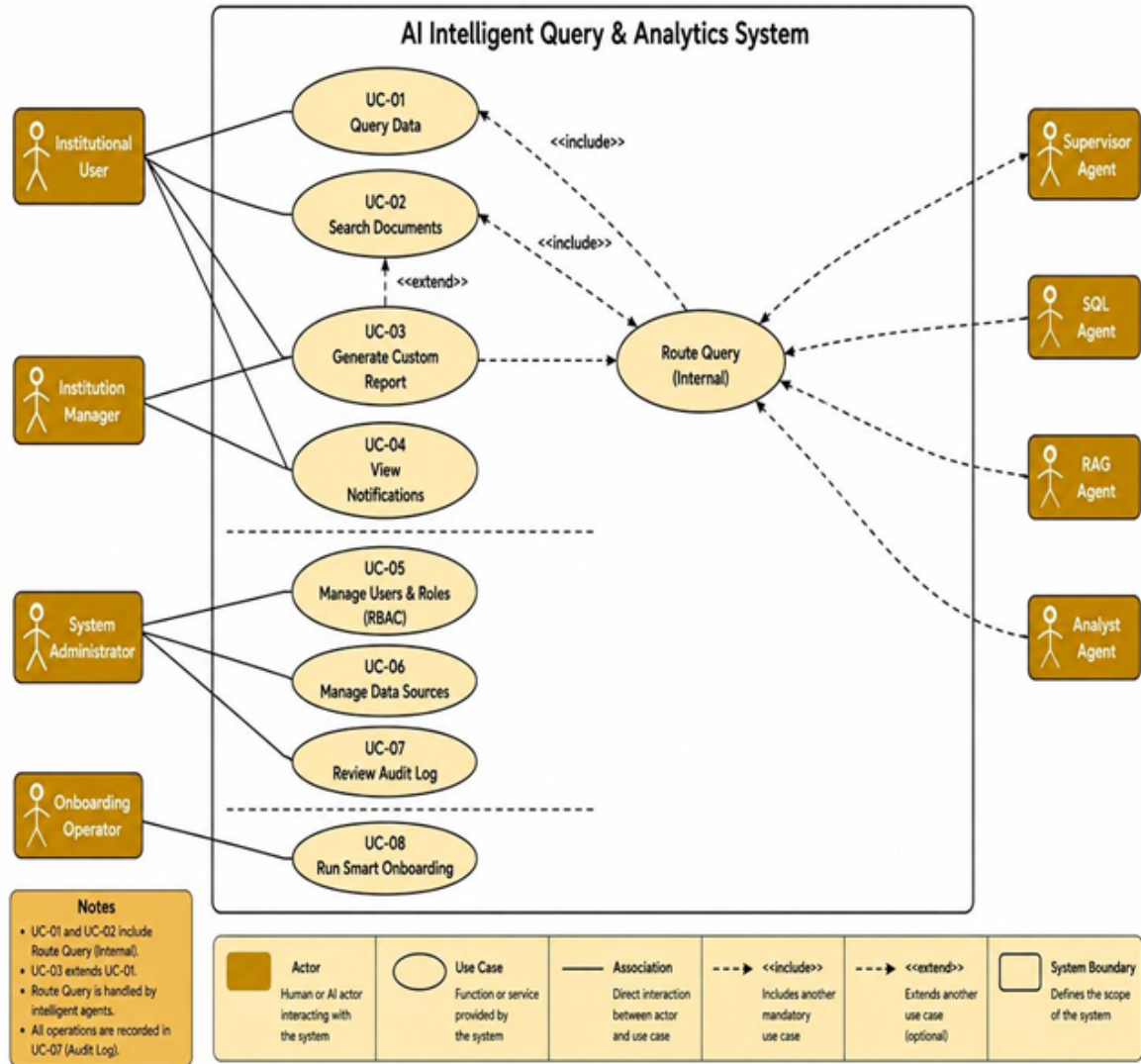
شكل 6-3: مخطط حالات استخدام نظام «بيان».
