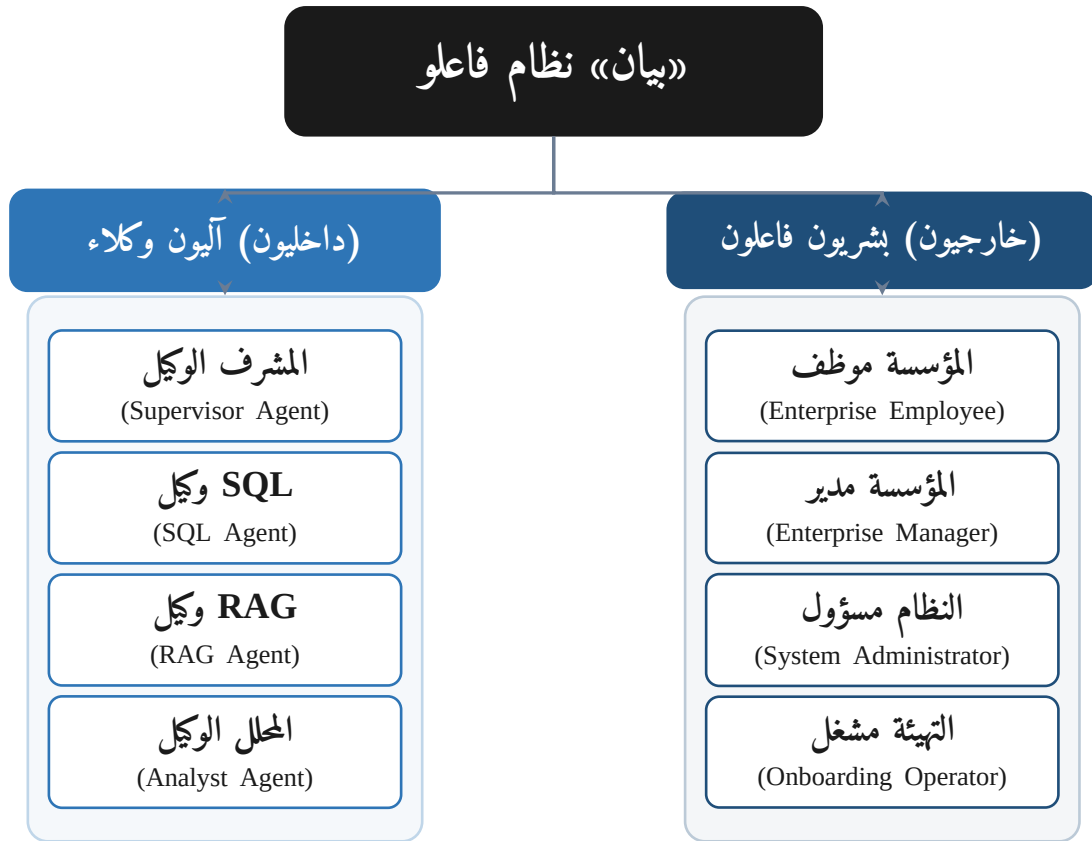
شكل 3-5: تصنيف فاعلي نظام «بيان» إلى فاعلين بشريين ووكلاء آليين.
